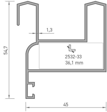
2023 BİNİLİ KASA PROFİLİ 0,790 kg/mt
