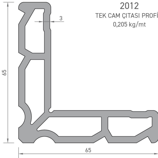
Kasa-Kanat Köşe Takoz Profili
