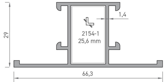
2024 ORTA KAYIT PROFİLİ 0,660 kg/mt
