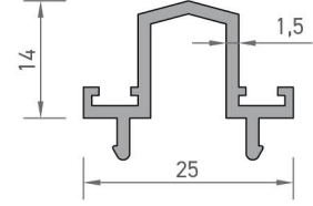
2028 KANAT BİRLEŞİM PROFİLİ 0,255 kg/mt
