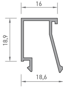
2012 TEK CAM ÇİTASI PROFİLİ 0,205 kg/mt
