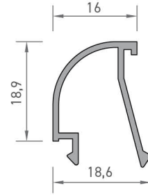
2013 OVAL ISI CAM ÇİTASI PROFİLİ 0,190 kg/mt
