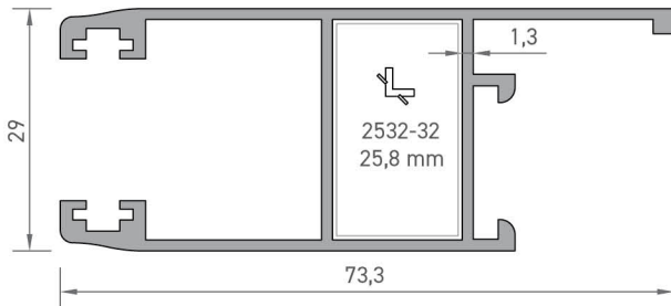
2021 KANAT PROFİLİ 0,815 kg/mt
