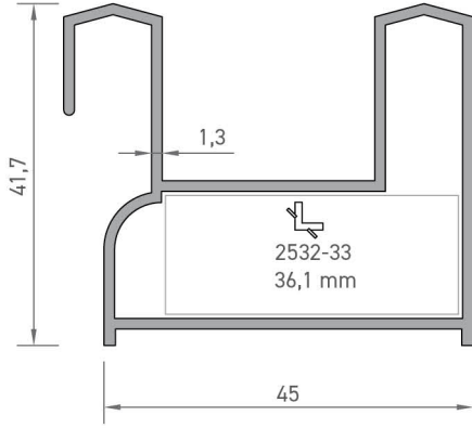
2020 KASA PROFİLİ 0,725 kg/mt
