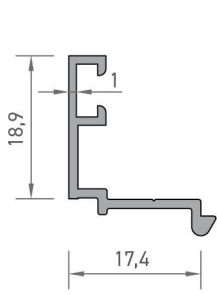
2027 KALIN CAM ÇİTASI TIRNAK ADAPTÖR PROFİLİ 0,170 kg/mt
