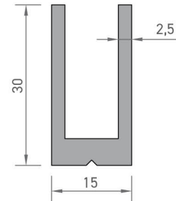
Kasa-Kanat Köşe Takoz Profili
