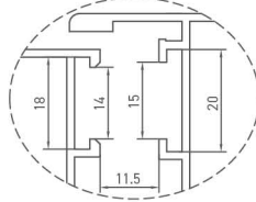
Euro Kanallı Kesit 1 Euro Groove Section 1
