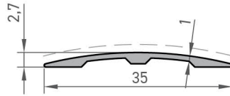
Kapı Altı Adaptör Profili Bottom Door Adapter Profile
