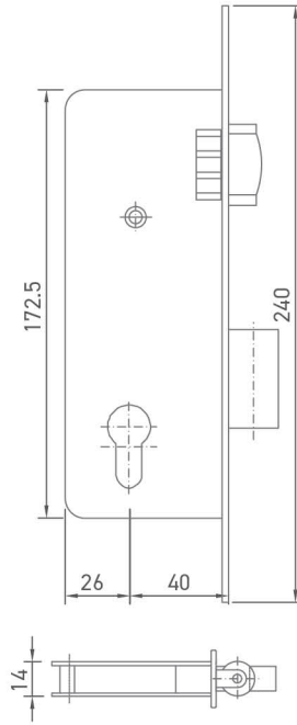
Geniş Kilit (Makaralı) Wide Type Lock (Roller)
