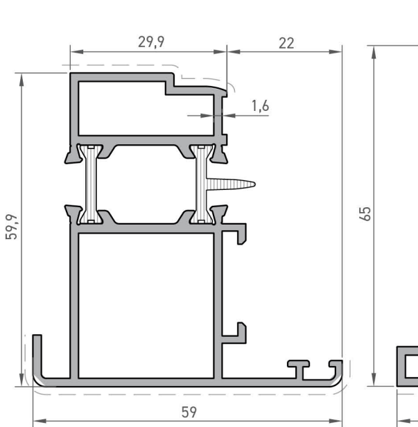
Pivot Adaptör Profili Pivot Adapter Profile
