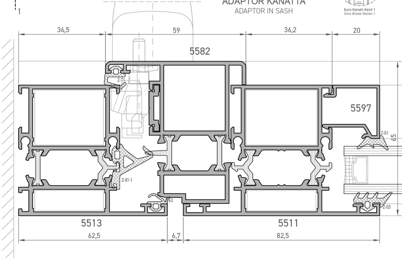
Pivot Açılır Pencere Pivot Opening Window
