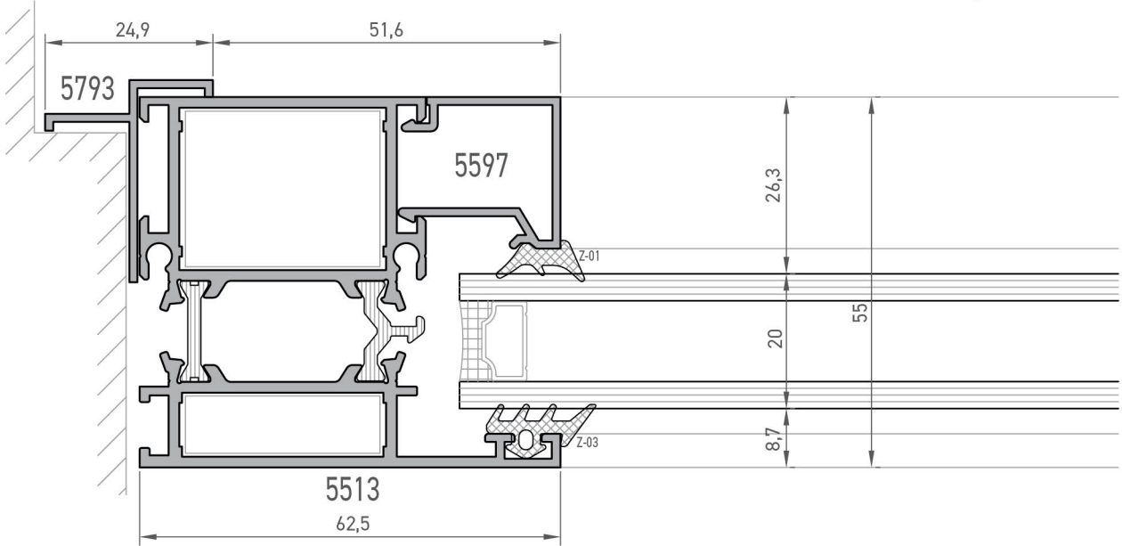
Euro Kanallı Kesit 1 euro groove section 1
