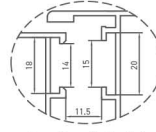
Euro Kanallı Kesit 1 Euro Groove Section 1
