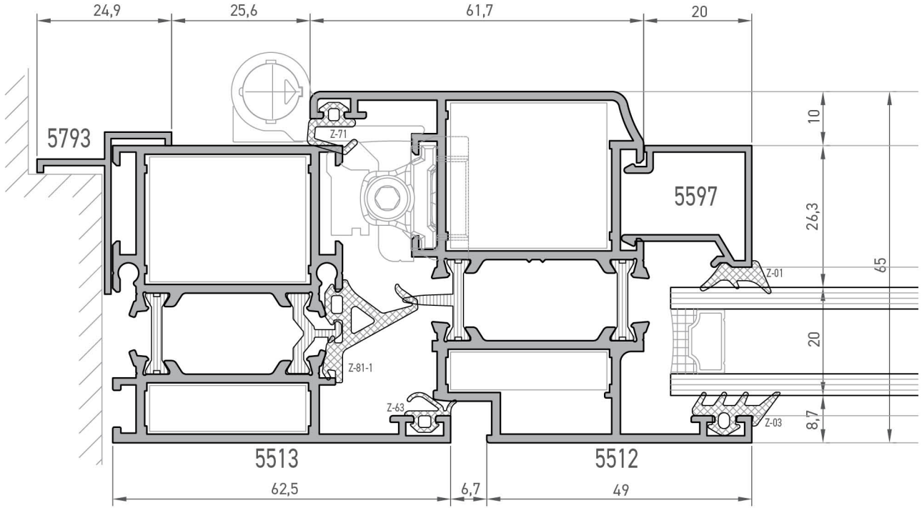
Euro Kanallı Kesit 1 euro groove section 1
