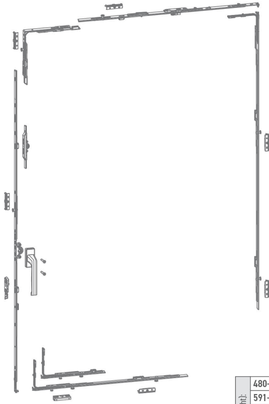
İçe Açılır Pencere Inward Opening Window
