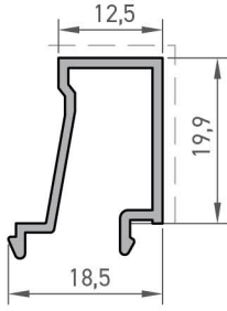
Cam Çıtası Profili Glazing Bead Profile
