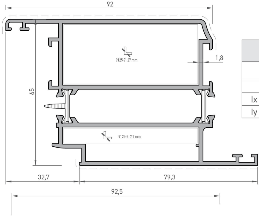
Kanat Profili (İçe Açılım) Sash Profile (Inward Opening)
