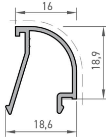
Cam Çıtası Profili Glazing Bead Profile
