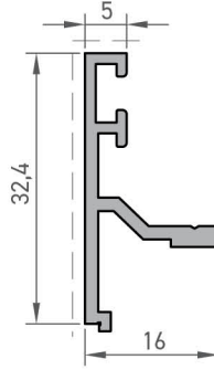
Adaptör Profili Adapter Profile
