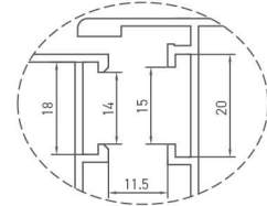
Euro Kanallı Kesit 1 Euro Groove Section 1
