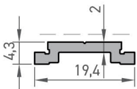
Tij Profili Rod Profile
