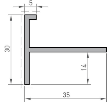
Kasa İç Çerçeve Profili Internal Frame Profile
