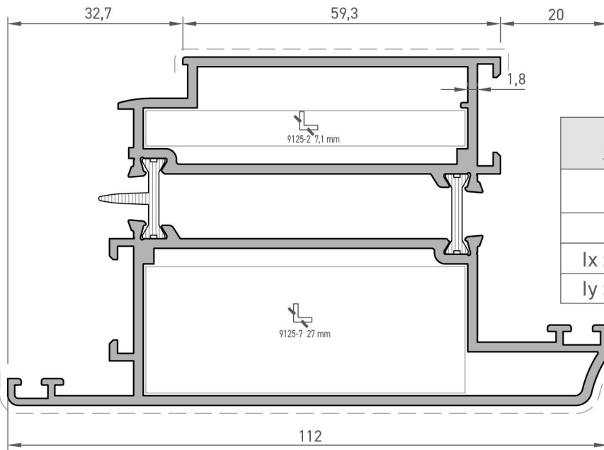
Kanat Profili (Dışa Açılım) Sash Profile (Outward Opening)
