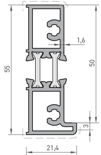
Eşik Profili Threshold Profile
