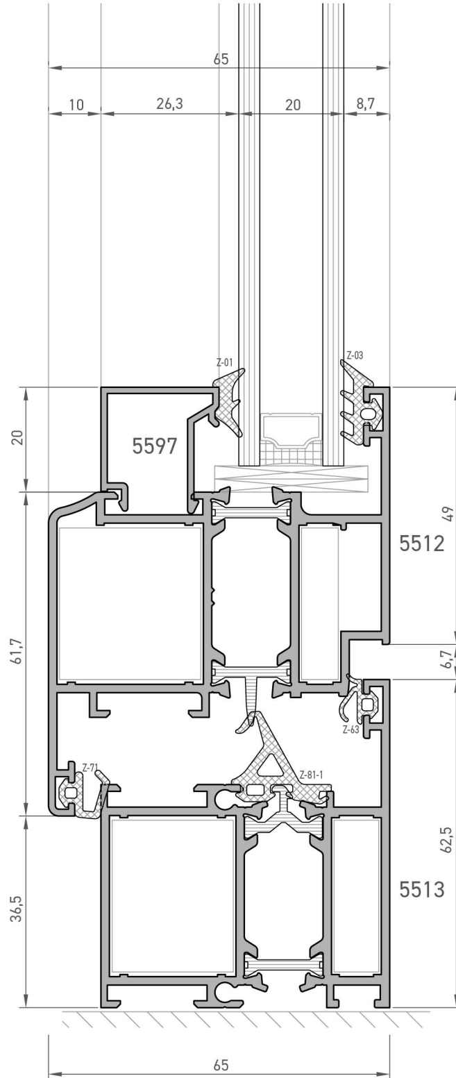
Euro Kanallı Kesit 1 Euro Groove Section 1
