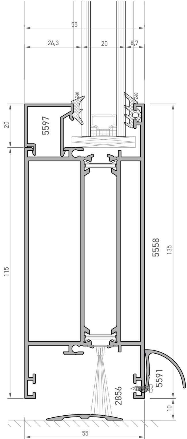
Euro Kanallı Kesit 1 Euro Groove Section 1
