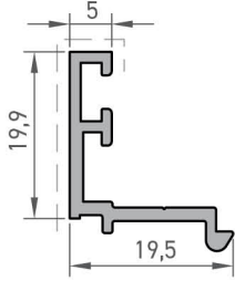
Adaptör Profili Adapter Profile
