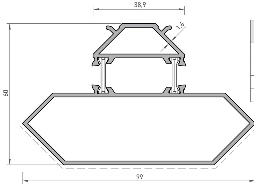
90° Köşe Dönüş Profili 90° Corner Return Profile
