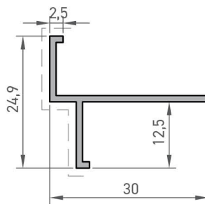
Kasa İç Çerçeve Profili Internal Frame Profile
