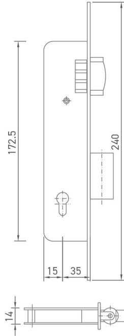
Geniş Kilit (Makaralı) Wide Type Lock (Roller)
