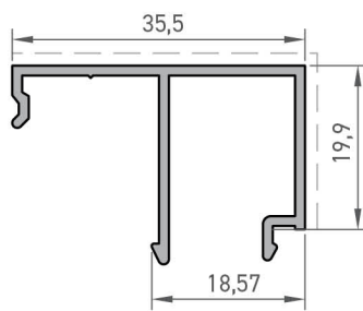
Cam Çıtası Profili Glazing Bead Profile
