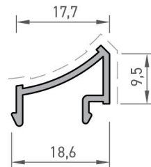
Köşe Dönüş Çıta Profili Corner Return Bead Profile
