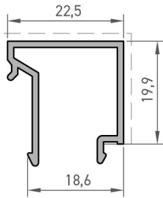
Cam Çıtası Profili Glazing Bead Profile
