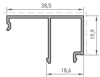
Cam Çıtası Profili Glazing Bead Profile
