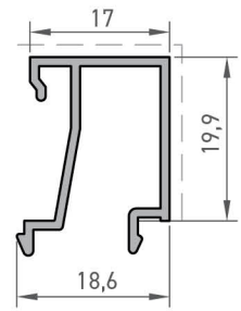
Cam Çıtası Profili Glazing Bead Profile
