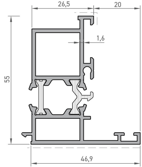
Kasa Adaptör Profili (Dışa Açılım) Frame Adapter Profile (Outward Opening)
