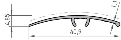
Kapı Altı Adaptör Profili Bottom Door Adapter Profile
