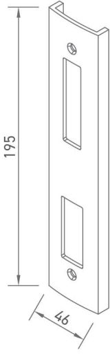
A051 KİLİT KARŞILIK (Dilli)
