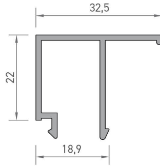
1995 CAM ÇİTASI PROFİLİ 0,345 kg/mt
