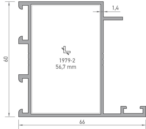
1981-14 KANAT PROFİLİ 1,060 kg/mt
