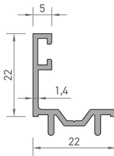
1990 TIRNAK PROFİLİ 0,255 kg/mt
