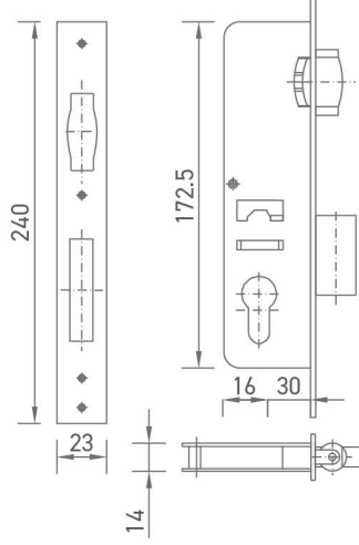
KT02-4 MAKARALI KİLİT
