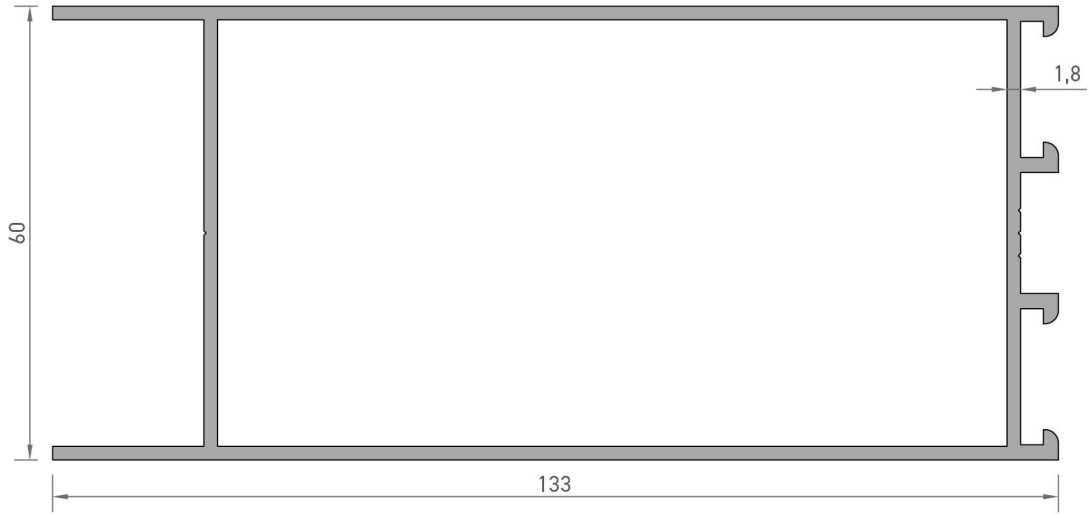
1982 ETEK PROFİLİ 1,945 kg/mt
