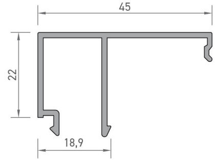
1974 ÇİTA PROFİLİ 0,410 kg/mt
