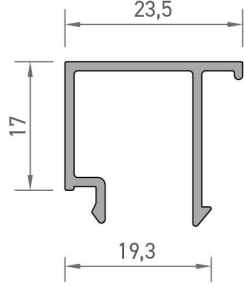
1986 KANAT ISI CAM ÇİTASI PROFİLİ 0,230 kg/mt
