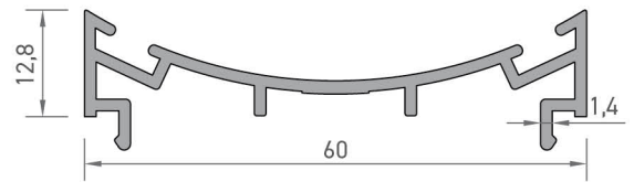
1989 ÇARPMA KAPI ADAPTÖR PROFİLİ 0,461 kg/mt
