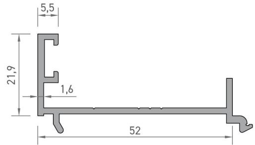
1987 KANAT ADAPTÖR PROFİLİ 0,462 kg/mt
