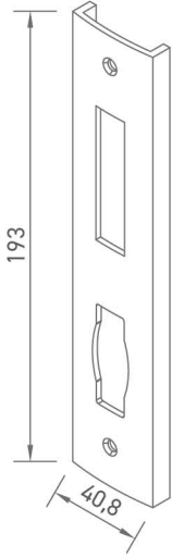
A051 KİLİT KARŞILIK (Makaralı)
