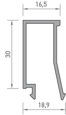
6135 KASA ISI CAM ÇİTASI PROFİLİ 0,342 kg/mt
