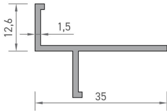
2529 FUGALI "T" PROFİLİ 0,245 kg/mt
