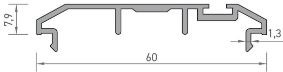
1988 ÇARPMA KAPI ADAPTÖR PROFİLİ 0,401 kg/mt
