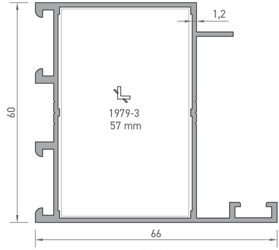
1998 GENİŞ KANAT PROFİLİ 0,940 kg/mt
