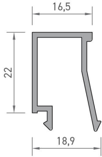
1985 KASA ISI CAM ÇİTASI PROFİLİ 0,285 kg/mt
