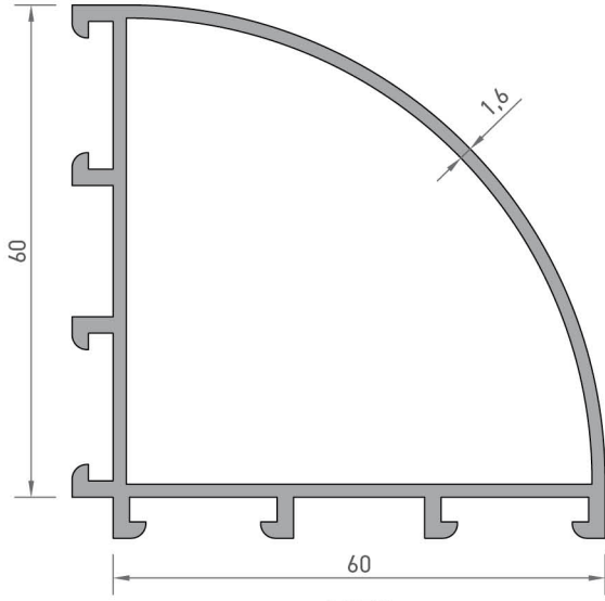
1983 KÖŞE PROFİLİ 1,195 kg/mt
