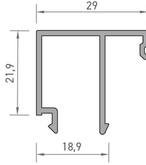
1997 CAM ÇİTASI PROFİLİ 0,350 kg/mt
