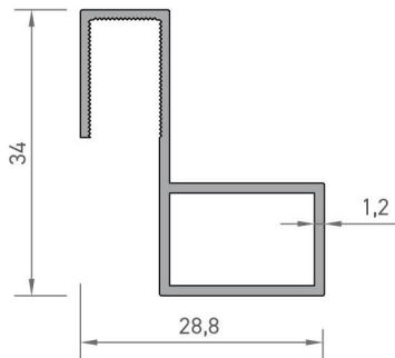
9283 AÇILIR KANAT KOL DİKME PROFİLİ 0,327 kg/mt
