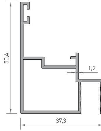
9284 KOL KARŞILIK PROFİLİ 0,536 kg/mt
