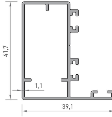
V.CB. 107 YAN KASA PROFİLİ 0,537 kg/mt
