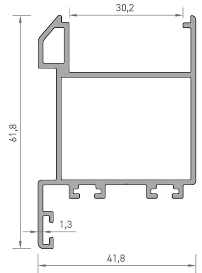
V.CB. 104 AÇILIR KANAT KOL DİKME PROFİLİ 0,830 kg/mt
