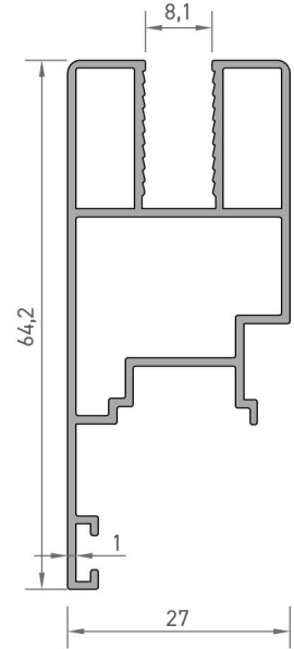
V.CB. 110 AÇILIR KANAT KOL DİKME PROFİLİ 0,620 kg/mt
