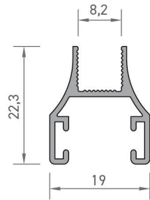
7320 ORTA ÇITA PROFİLİ 0,210 kg/mt
