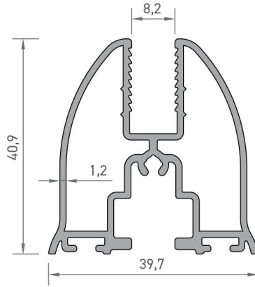
6272 KANAT PROFİLİ 0,790 kg/mt
