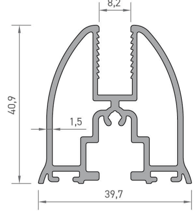
4221 KANAT PROFİLİ 0,905 kg/mt
