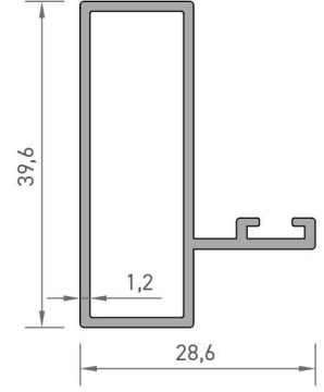
6271 YAN KASA PROFİLİ 0,410 kg/mt
