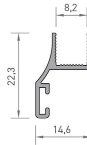
7321 ORTA ÇITA PROFİLİ 0,140 kg/mt
