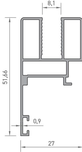
V.CB. 111 AÇILIR KANAT BİRLEŞİM PROFİLİ 0,526 kg/mt
