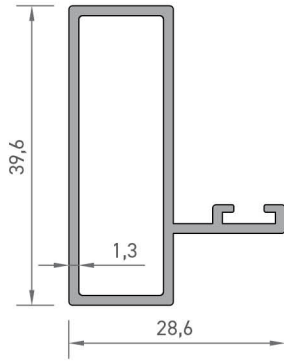
4223 YAN KASA PROFİLİ 0,435 kg/mt
