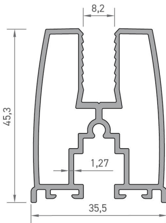
V.CB. 108 KANAT ALT-ÜST PROFİLİ 0,850 kg/mt
