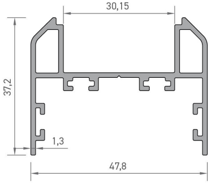
V.CB. 106 KANAT BİRLEŞİM PROFİLİ 0,680 kg/mt
