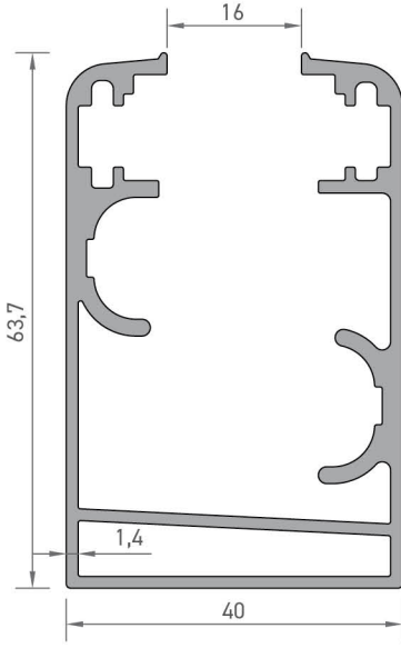
6273 KASA PROFİLİ 1,250 kg/mt
