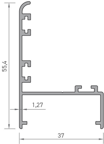
V.CB.102 90° DÖNÜŞ PROFİLİ 0,493 kg/mt
