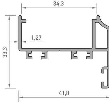
V.CB. 103 AÇILIR KANAT BİRLEŞİM PROFİLİ 0,474 kg/mt
