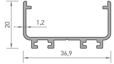
V.CB. 105 GEÇİŞ PROFİLİ 0,301 kg/mt
