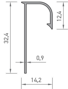
2891 SERAMİK DÖNÜŞ PROFİLİ 0,137 kg/mt
