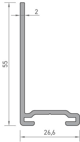
7461 TAŞIYICI "L" PROFİLİ 0,475 kg/mt
