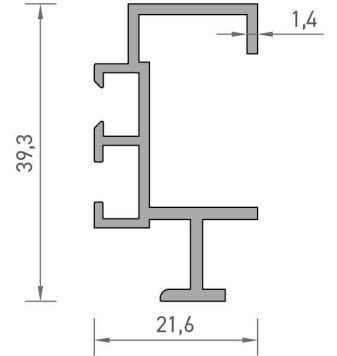
2864 KOMPOZİT KASET PROFİLİ 0,415 kg/mt
