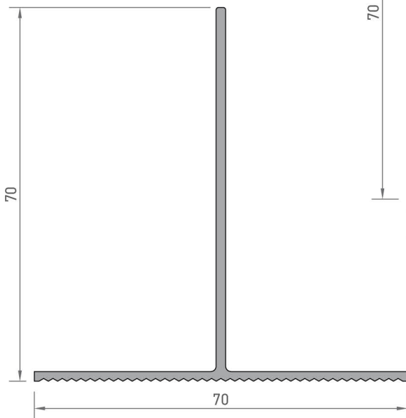
9280 ÜST KLİPS PROFİLİ 0,629 kg/mt
