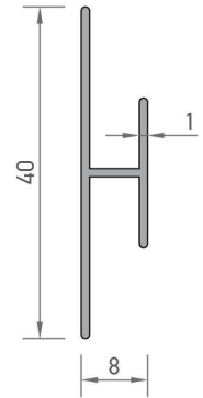
7288 KOMPOZİT "H" PROFİLİ 0,175 kg/mt
