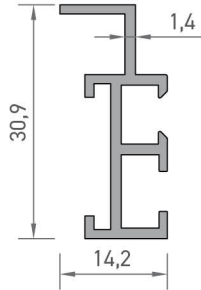
3251 KOMPOZİT KASET PROFİLİ (4 mm) 0,270 kg/mt
