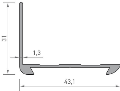
2089 SERAMİK PROFİLİ 0,296 kg/mt
