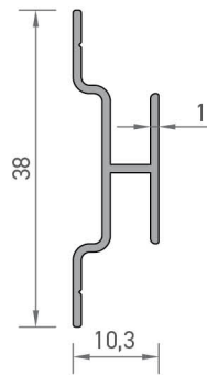
6496 KOMPOZİT "H" PROFİLİ 0,175 kg/mt
