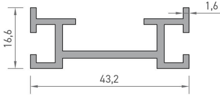
4720 KOMPOZİT BAĞLANTI PROFİLİ 0,500 kg/mt
