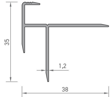
2855 HALI PROFİLİ 0,275 kg/mt
