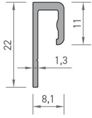
5423 SERAMİK DÖNÜŞ PROFİLİ 0,155 kg/mt
