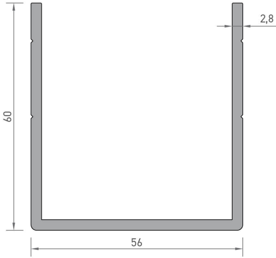
3451 KOMPOZİT "U" PROFİLİ 1,290 kg/mt
