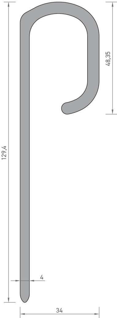
4997 SERAMİK DÖNÜŞ PROFİLİ 2,355 kg/mt
