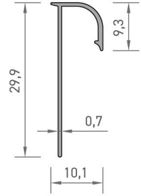
2264 SERAMİK DÖNÜŞ PROFİLİ 0,91 kg/mt
