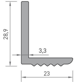
3927 SERAMİK PROFİLİ 0,411 kg/mt
