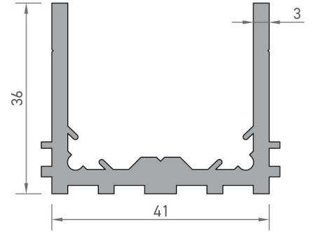
3493 KOMPOZİT BAĞLANTI PROFİLİ 1,050 kg/mt
