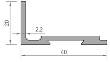
3409 SERAMİK PROFİLİ 0,390 kg/mt
