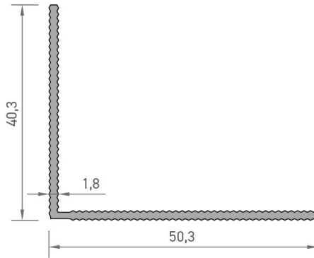
7921 SERAMİK PROFİLİ 0,357 kg/mt
