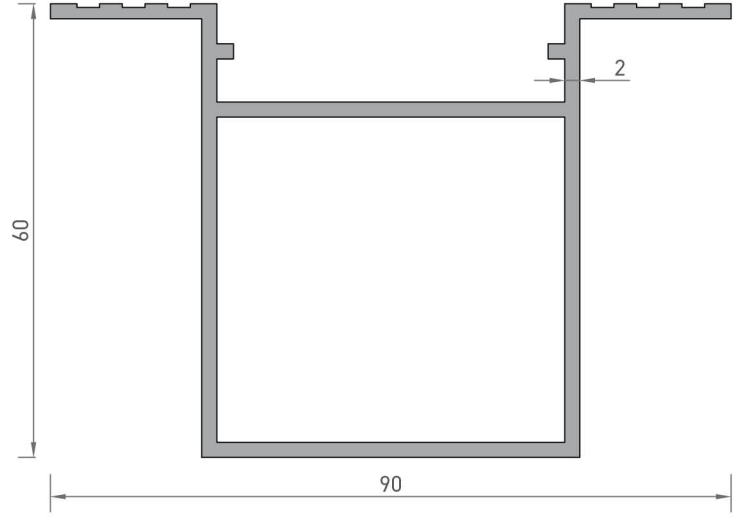
3452 KOMPOZİT KASA PROFİLİ 1,365 kg/mt
