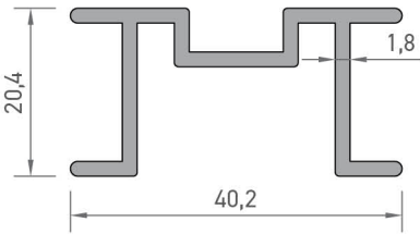
4934 KOMPOZİT LEVHA DÖNÜŞ PROFİLİ 0,490 kg/mt
