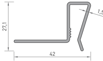
2224 KOMPOZİT LEVHA DÖNÜŞ PROFİLİ 0,365 kg/mt
