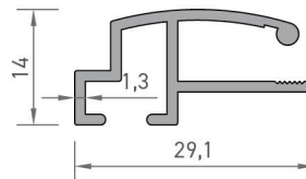
2805 İLÂN ÇERÇEVE PROFİLİ 0,261 kg/mt
