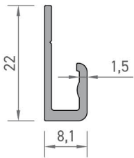
2266 KOMPOZİT "U" PROFİLİ 0,155 kg/mt
