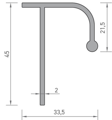
4847 SERAMİK DÖNÜŞ PROFİLİ 0,518 kg/mt
