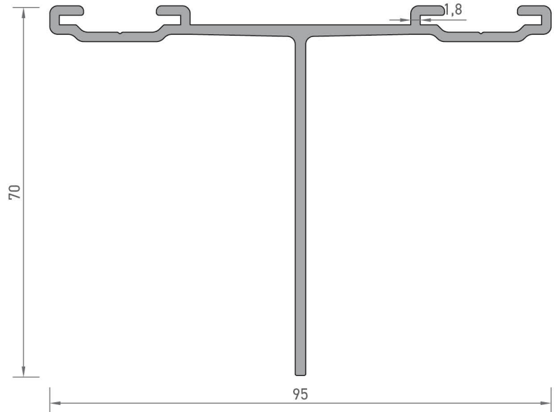
3818 TAŞIYICI "T" PROFİLİ 0,999 kg/mt
