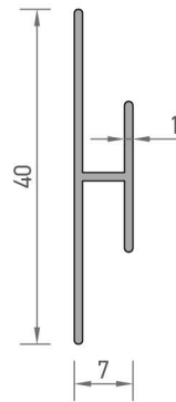
4117 KOMPOZİT "H" PROFİLİ 0,170 kg/mt
