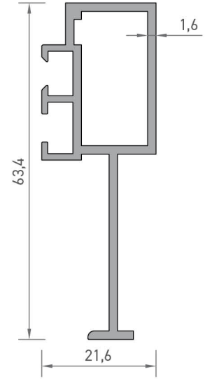
2297 KOMPOZİTKASET DUVAR BİRLEŞİM PROFİLİ 0,635 kg/mt
