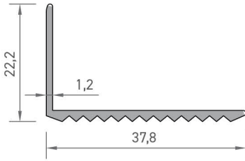
2088 SERAMİK PROFİLİ 0,225 kg/mt
