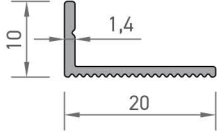
7604 SERAMİK PROFİLİ 0,097 kg/mt
