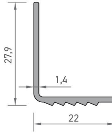
2256 SERAMİK PROFİLİ 0,200 kg/mt
