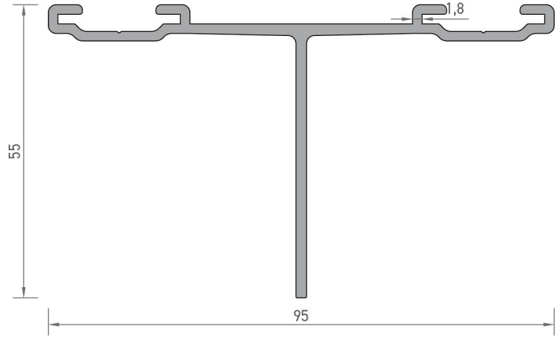
3817 TAŞIYICI "T" PROFİLİ 0,920 kg/mt
