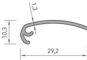
2806 İLÂN ÇERÇEVE PROFİLİ 0,147 kg/mt
