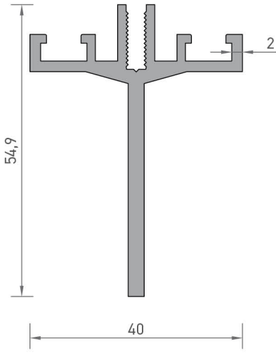
3250 KOMPOZİT KASA PROFİLİ 0,815 kg/mt
