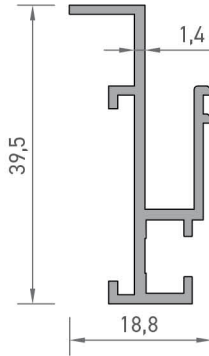
3258 KOMPOZİT KASET PROFİLİ (6 mm) 0,340 kg/mt
