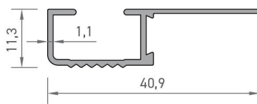
2398 BASAMAK PROFİLİ 0,192 kg/mt
