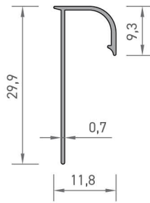
2265 SERAMİK DÖNÜŞ PROFİLİ 0,95 kg/mt
