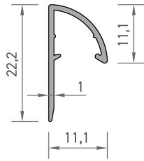
3222 SERAMİK DÖNÜŞ PROFİLİ 0,110 kg/mt
