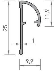
2708 SERAMİK DÖNÜŞ PROFİLİ 0,130 kg/mt
