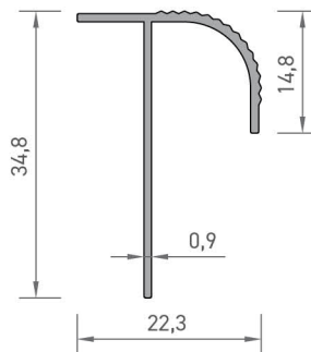
2890 SERAMİK DÖNÜŞ PROFİLİ 0,177 kg/mt
