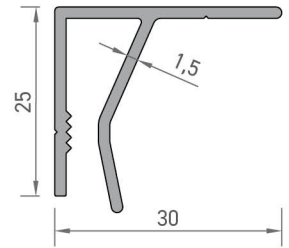
5425 KOMPOZİT LEVHA DÖNÜŞ PROFİLİ 0,335 kg/mt
