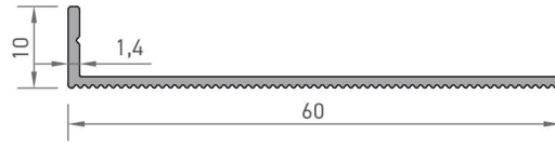
7842 SERAMİK PROFİLİ 0,227 kg/mt
