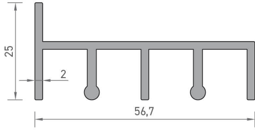
2728 SOĞUTUCU PROFİLİ 0,755 kg/mt
