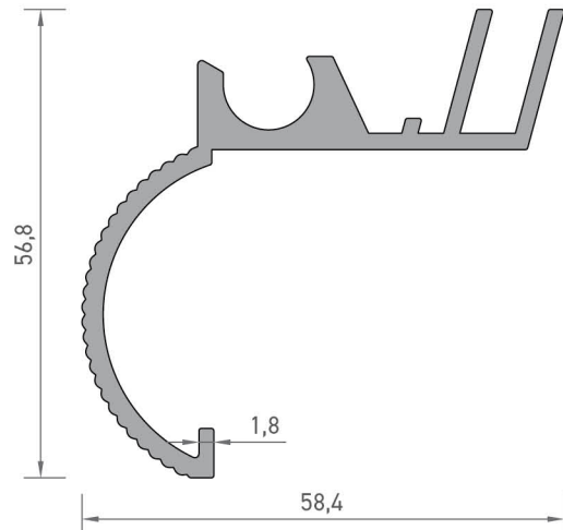
2730 SOĞUTUCU PROFİLİ 0,980 kg/mt
