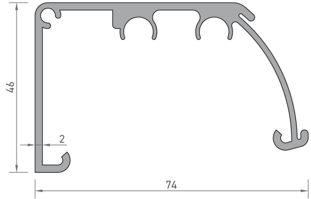
2727 SOĞUTUCU PROFİLİ 1,075 kg/mt
