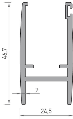
2729 SOĞUTUCU PROFİLİ 0,695 kg/mt
