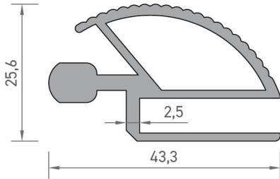
2726 SOĞUTUCU PROFİLİ 0,795 kg/mt
