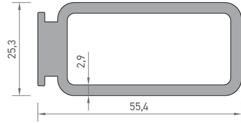
2731 SOĞUTUCU PROFİLİ 1,282 kg/mt
