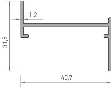
3814 MENFEZ KASA PROFİLİ 0,320 kg/mt
