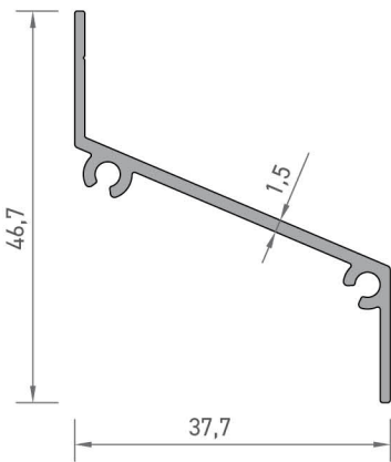
3815 MENFEZ YAPRAK PROFİLİ 0,315 kg/mt
