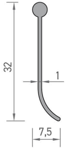
2245 MENFEZ YAPRAK PROFİLİ 0,115 kg/mt
