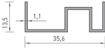
2435 PANJUR PROFİLİ 0,245 kg/mt
