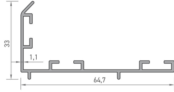
2096 MENFEZ KASA PROFİLİ 0,435 kg/mt
