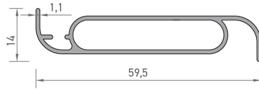
2434 MENFEZ YAPRAK PROFİLİ 0,390 kg/mt
