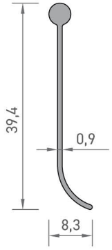
4537 MENFEZ YAPRAK PROFİLİ 0,130 kg/mt
