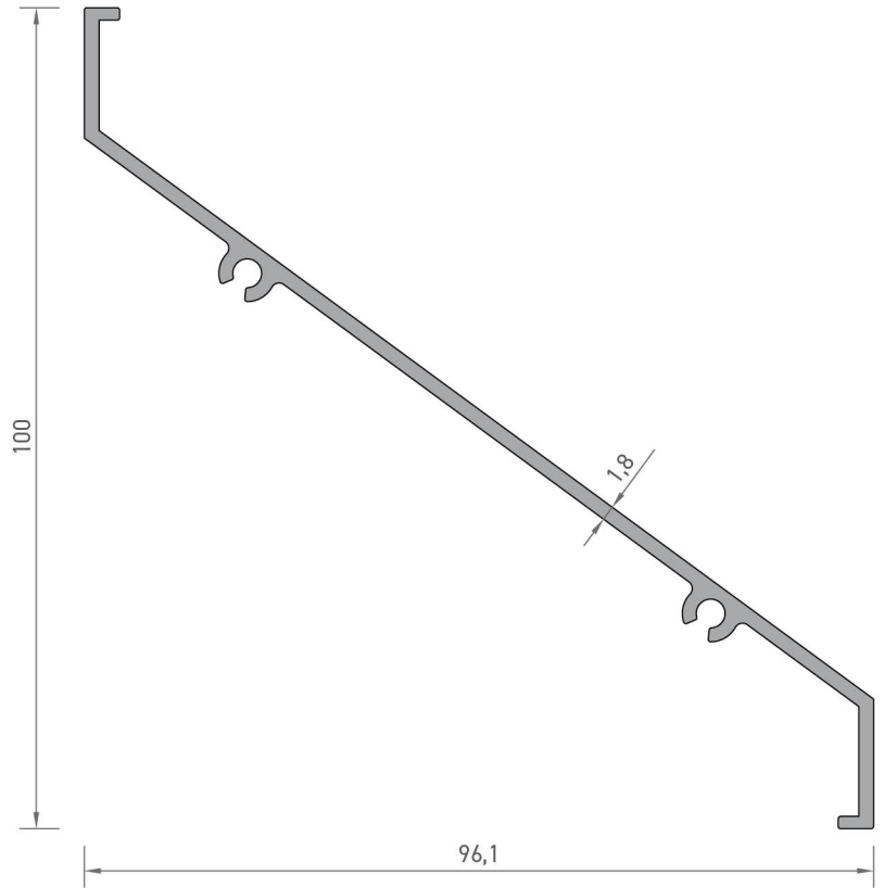
8808 MENFEZ YAPRAK PROFİLİ 0,825 kg/mt
