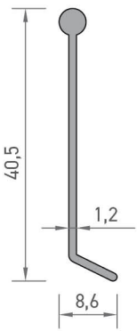
2053 MENFEZ YAPRAK PROFİLİ 0,160 kg/mt
