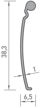
2042 MENFEZ YAPRAK PROFİLİ 0,140 kg/mt
