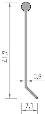
2048 MENFEZ YAPRAK PROFİLİ 0,131 kg/mt
