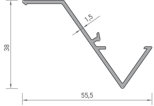
7496 MENFEZ YAPRAK PROFİLİ 0,370 kg/mt
