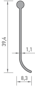
2753 MENFEZ YAPRAK PROFİLİ 0,150 kg/mt
