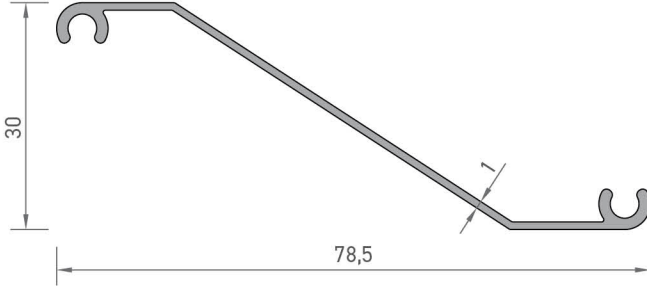
9003 MENFEZ YAPRAK PROFİLİ 0,306 kg/mt
