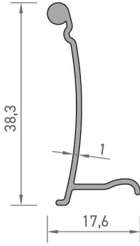
2044 MENFEZ YAPRAK PROFİLİ 0,177 kg/mt
