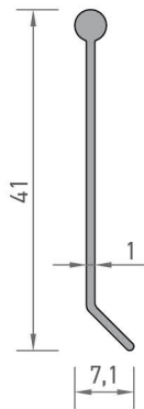
3103 MENFEZ YAPRAK PROFİLİ 0,140 kg/mt
