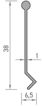
2084 MENFEZ YAPRAK PROFİLİ 0,130 kg/mt
