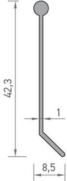
2240 MENFEZ YAPRAK PROFİLİ 0,150 kg/mt
