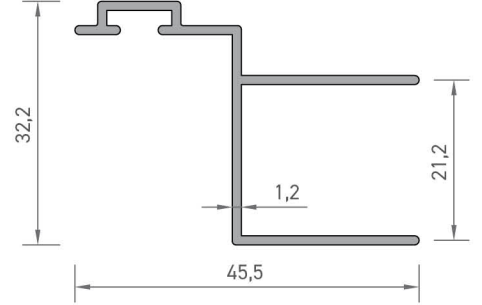
3100 KAPI KARŞILIK PROFİLİ 0,345 kg/mt
