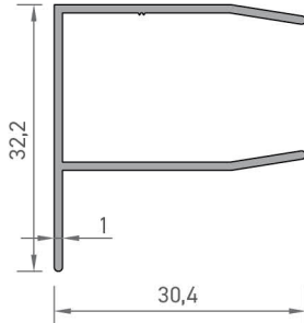
7390 KAPI KARŞILIK PROFİLİ 0,245 kg/mt
