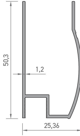
7568 CAM PROFİLİ 0,410 kg/mt
