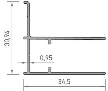
2373 DUVAR DİKMESİ PROFİLİ 0,274 kg/mt
