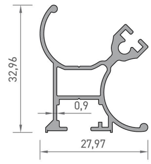
8509 KÖŞE KİRİŞLİ DİKME PROFİLİ 0,374 kg/mt
