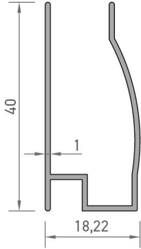
7569 CAM PROFİLİ 0,276 kg/mt
