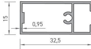
2365 ASKILIK PROFİLİ 0,292 kg/mt
