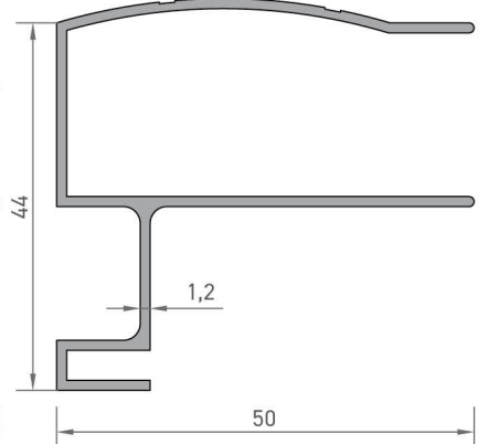
7565 KAPI KARŞILIK PROFİLİ 0,530 kg/mt
