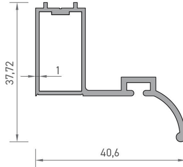
2366 KISA KAPI KARŞILIK PROFİLİ 0,341 kg/mt
