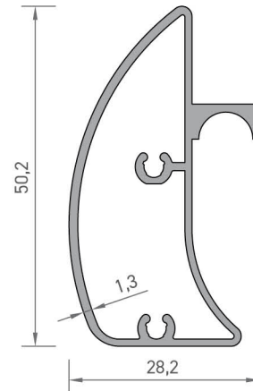
3864 RAY PROFİLİ 0,536 kg/mt
