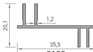
9182 KAPI KARŞILIK PROFİLİ 0,242 kg/mt
