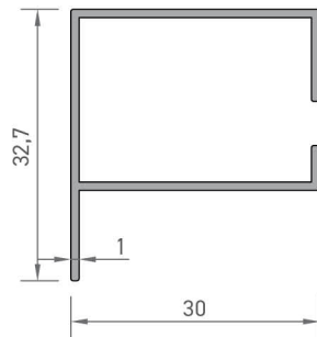
8587 KAPI KARŞILIK PROFİLİ 0,285 kg/mt
