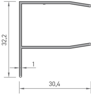
7390 KAPI KARŞILIK PROFİLİ 0,245 kg/mt
