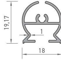
2362 ORTA DİKME PROFİLİ 0,221 kg/mt
