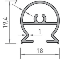
2360 ÖN DİKME PROFİLİ 0,230 kg/mt
