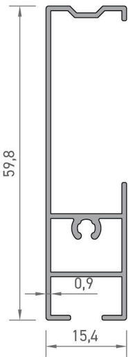
8510 FİTİLLİ ASKILIK PROFİLİ 0,401 kg/mt
