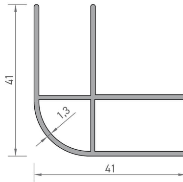
2384 AÇILI BAĞLI DİKMES PROFİLİ 0,521 kg/mt
