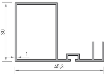
8589 KAPI KARŞILIK PROFİLİ 0,405 kg/mt
