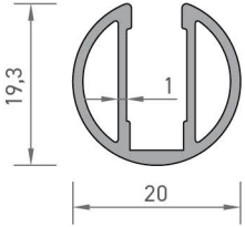
3096 CAM KABİN PROFİLİ 0,277 kg/mt
