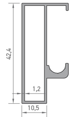
6302 İÇ RAY PROFİLİ 0,415 kg/mt
