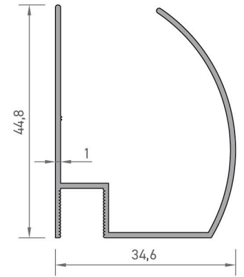
7389 CAM PROFİLİ 0,355 kg/mt
