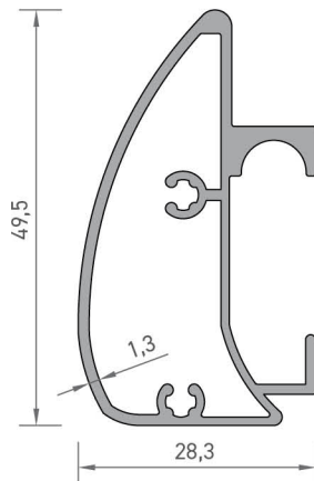
8119 RAY PROFİLİ 0,602 kg/mt
