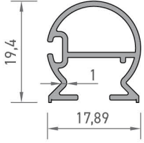
2361 ARKA DİKME PROFİLİ 0,217 kg/mt
