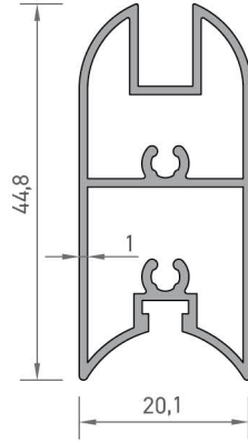
3095 CAM KABİN PROFİLİ 0,519 kg/mt
