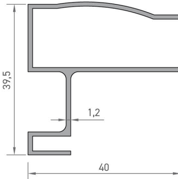
7566 KAPI KARŞILIK PROFİLİ 0,425 kg/mt
