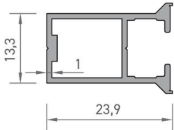
2370 ARKA SABİT PROFİLİ 0,241 kg/mt
