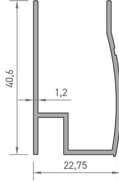
6366 CAM PROFİLİ 0,360 kg/mt
