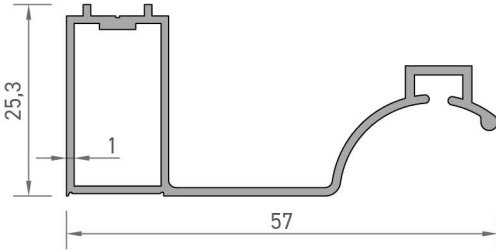
2367 UZUN KAPI KARŞILIK PROFİLİ 0,406 kg/mt
