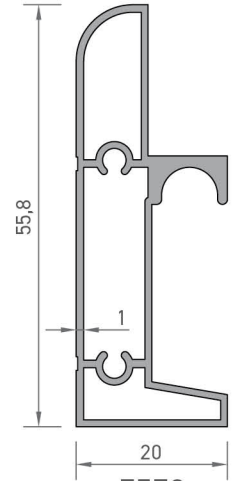
7570 RAY PROFİLİ 0,518 kg/mt
