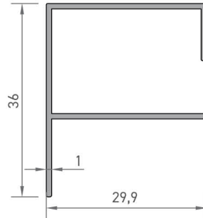
6303 KAPI KARŞILIK PROFİLİ 0,280 kg/mt
