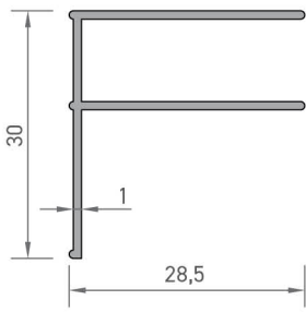
7567 KAPI KARŞILIK PROFİLİ 0,230 kg/mt
