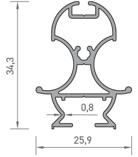
8508 ORTA DİKME PROFİLİ 0,374 kg/mt
