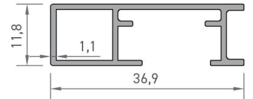
2372 JAKUZİ İÇ RAY PROFİLİ 0,267 kg/mt
