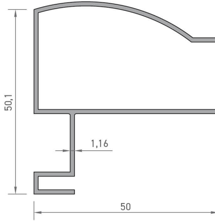
3863A KAPI KARŞILIK PROFİLİ 0,534 kg/mt
