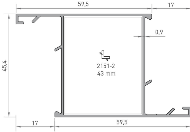
6096 GENİŞ KANAT PROFİLİ 0,603 kg/mt
