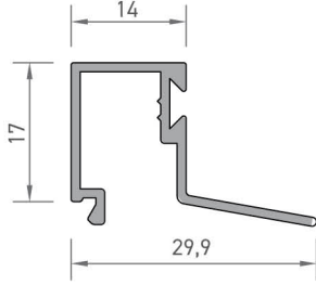
2105 ISI CAM ÇİTASI PROFİLİ 0,230 kg/mt
