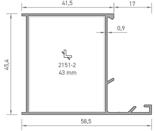
6094 GENİŞ KASA PROFİLİ 0,507 kg/mt
