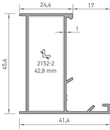
2180 DAR KASA PROFİLİ 0,460 kg/mt
