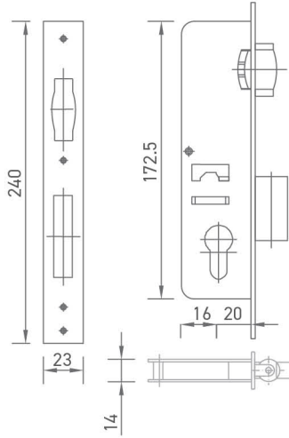
KT01-6 MAKARALI KİLİT
