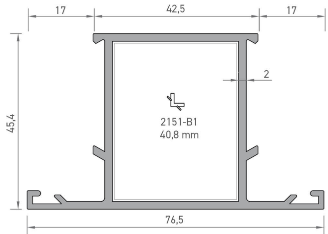
2186 GENİŞ ORTA KAYIT PROFİLİ 1,165 kg/mt
