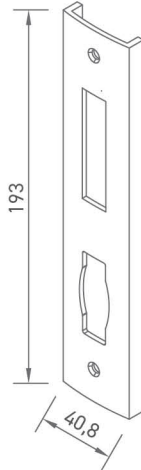
A050 ALDOKS KİLİT KARŞILIK (MAKARALI)
