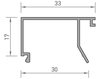
4178 TEK CAM ÇİTASI PROFİLİ 0,220 kg/mt
