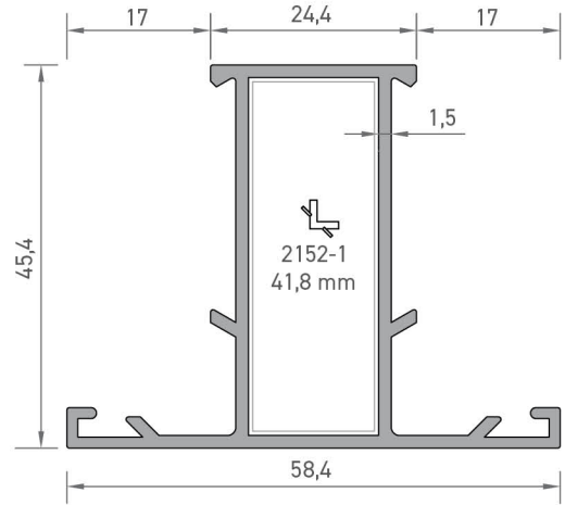
2202 DAR ORTA KAYIT PROFİLİ 0,770 kg/mt
