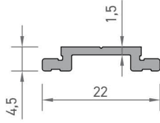
2640 TİJ ÇUBUK DIŞ PROFİLİ 0,120 kg/mt
