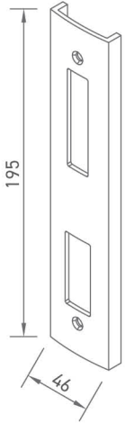
A050 ALDOKS KİLİT KARŞILIK (DİLLİ)
