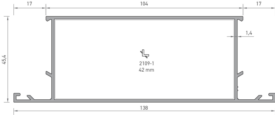
2110 BAZA ORTA KAYIT PROFİLİ 1,385 kg/mt
