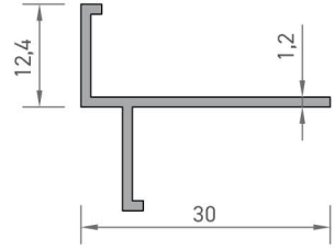
2530 FUGALI T 0,185 kg/mt
