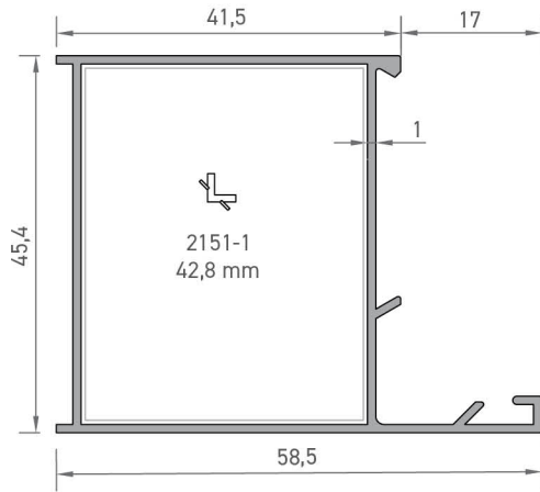
2183 GENİŞ KASA PROFİLİ 0,550 kg/mt
