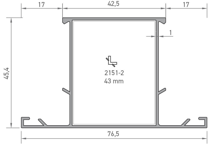
2182 GENİŞ ORTA KAYIT PROFİLİ 0,645 kg/mt
