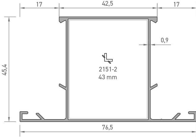
6095 GENİŞ ORTA KAYIT PROFİLİ 0,603 kg/mt
