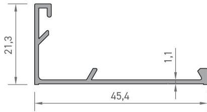
2121 ALDOKS TIRNAK PROFİLİ 0,245 kg/mt
