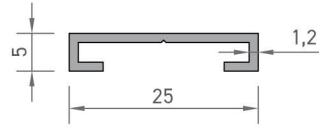
2639 TİJ ÇUBUK DIŞ PROFİLİ 0,130 kg/mt
