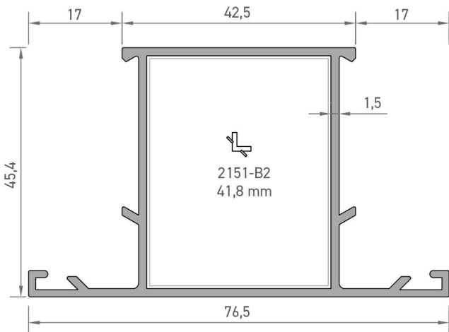
2205 GENİŞ ORTA KAYIT PROFİLİ 0,920 kg/mt
