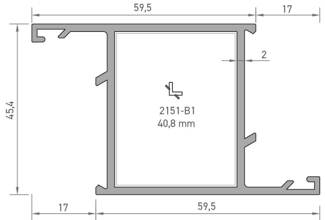
2187 GENİŞ KANAT PROFİLİ 1,165 kg/mt
