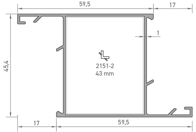
2181 GENİŞ KANAT PROFİLİ 0,645 kg/mt
