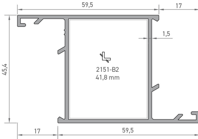
2204 GENİŞ KANAT PROFİLİ 0,925 kg/mt
