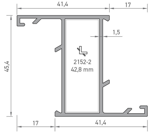
2201 DAR KANAT PROFİLİ 0,770 kg/mt
