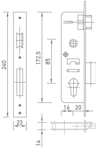
KT01-5 DİLLİ KİLİT
