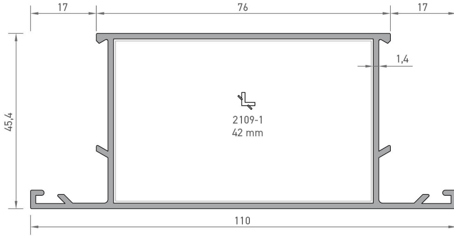
2207 BAZA ORTA KAYIT PROFİLİ 1,160 kg/mt
