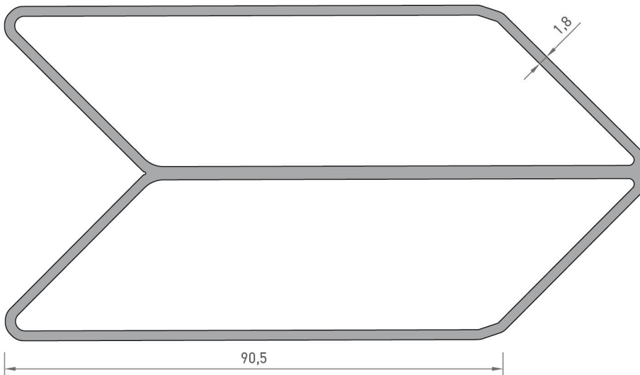
2110 BAZA ORTA KAYIT PROFİLİ 1,385 kg/mt
