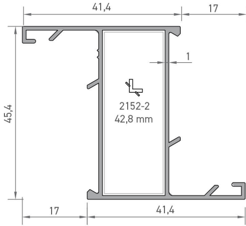
2178 DAR KANAT PROFİLİ 0,550 kg/mt
