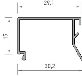
2104 TEK CAM ÇİTASI PROFİLİ 0,190 kg/mt
