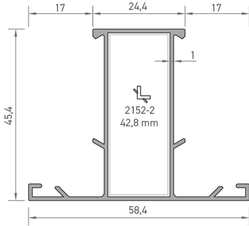
2179 DAR ORTA KAYIT PROFİLİ 0,550 kg/mt
