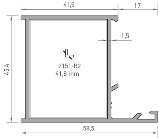
2206 GENİŞ KASA PROFİLİ 0,800 kg/mt
