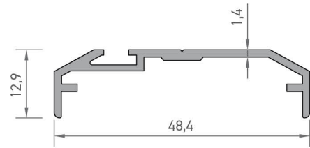
2175 ÇARPMA KAPI ADAPTÖR PROFİLİ 0,310 kg/mt
