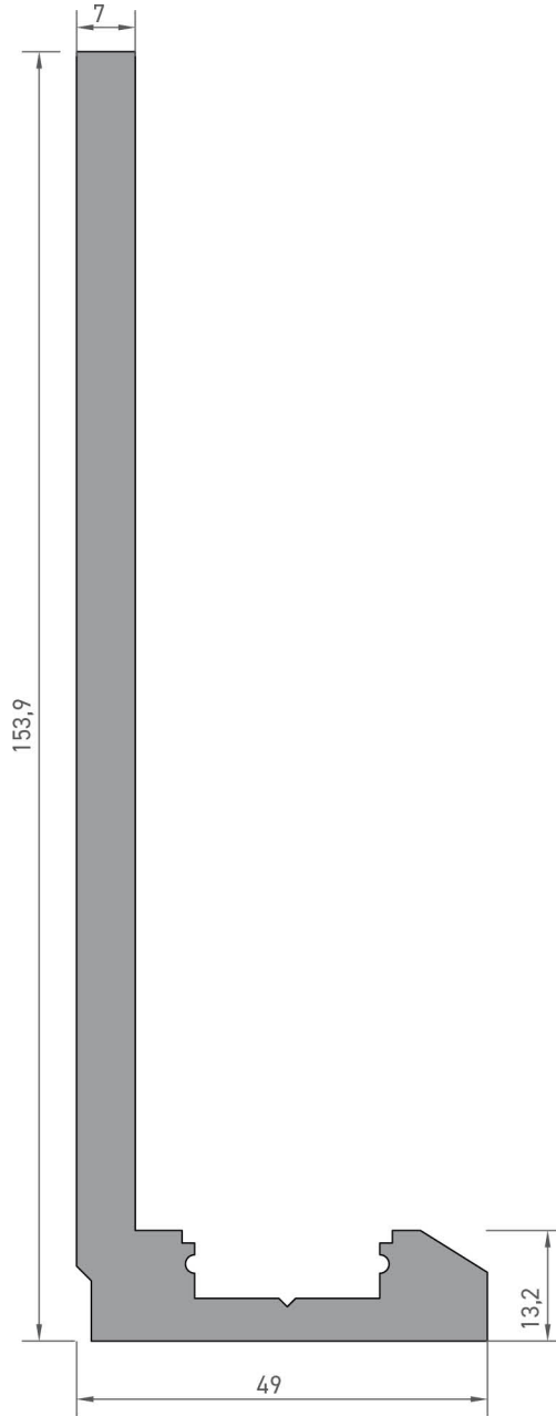
5490 ANKRAJ PROFİLİ 3,820 kg/mt Jx : 351,85 cm 4 Jy : 16,24 cm 4
