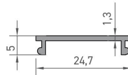
5489 ANKRAJ KAPAK PROFİLİ 0,115 kg/mt
