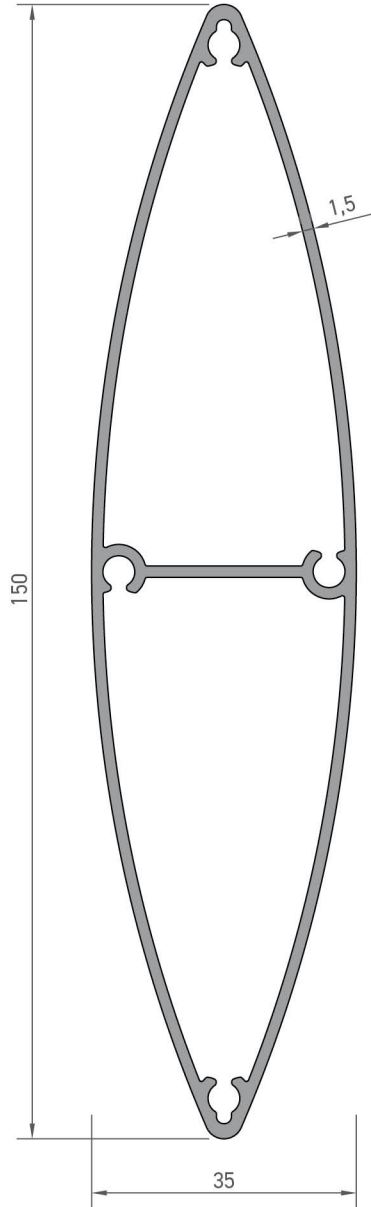
3762 GÜNEŞ KIRICI PROFİLİ 1,475 kg/mt Jx : 97,05 cm 4 Jy : 7,75 cm 4
