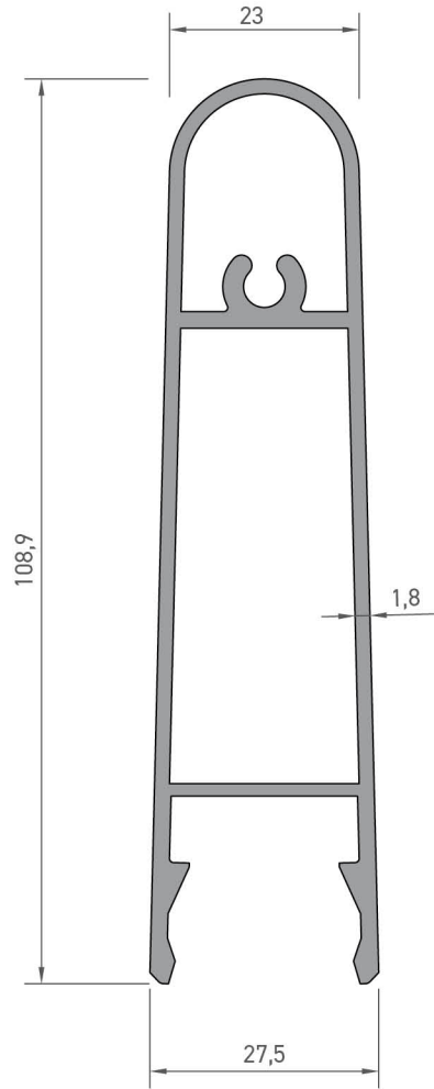
5499 GÜNEŞ KIRICI YAPRAK PROFİLİ 1,500 kg/mt Jx : 58,61 cm 4 Jy : 5,85 cm 4
