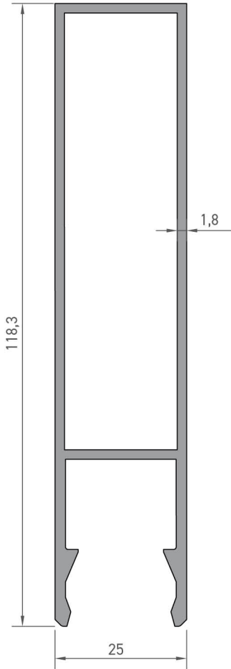
5494 KASA UÇ PROFİLİ (25'LİK) 1,455 kg/mt Jx : 72,83 cm 4 Jy : 6,40 cm 4
