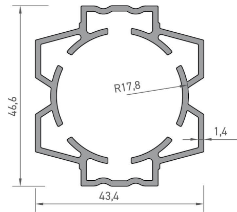
4723 ORTA BAĞLANTI PROFİLİ 0,965 kg/mt
