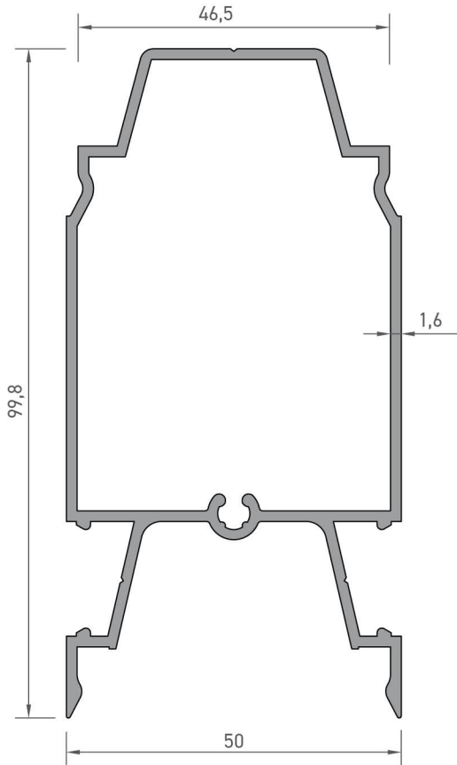
2490 ORTA BAĞLANTI PROFİLİ 1,355 kg/mt Jx : 45,74 cm 4 Jy : 18,63 cm 4
