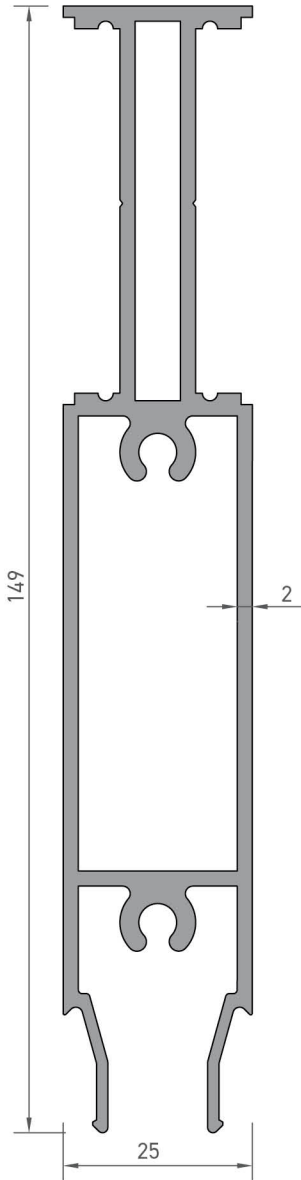
5493 KASA ARKA ROFİLİ (25'LİK) 2,250 kg/mt Jx : 153,31 cm 4 Jy : 5,73 cm 4
