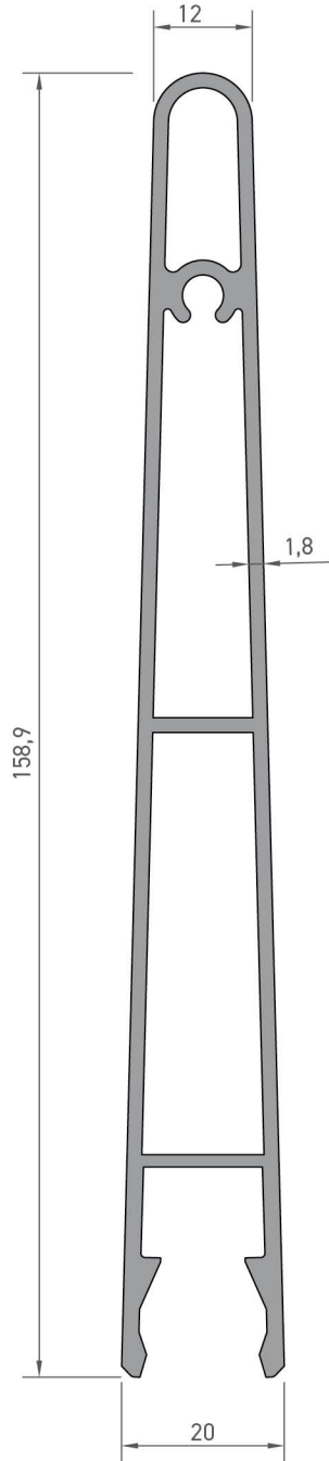
5498 GÜNEŞ KIRICI YAPRAK PROFİLİ 1,880 kg/mt Jx : 3,13 cm 4 Jy : 156,41 cm 4
