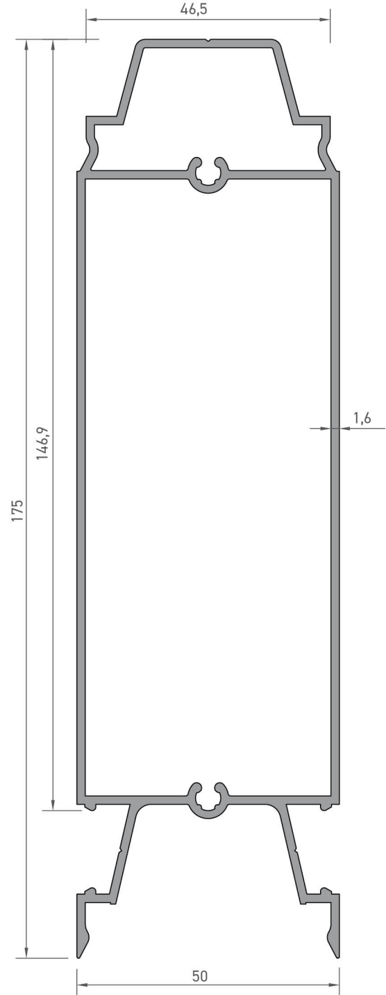
2491 ORTA BAĞLANTI PROFİLİ 2,245 kg/mt Jx : 260,80 cm 4 Jy : 34,00 cm 4
