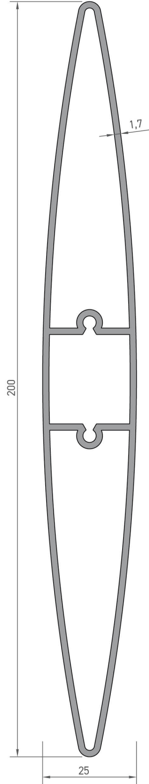
4399 GÜNEŞ KIRICI PROFİLİ 2,140 kg/mt Jx : 233,67 cm 4 Jy : 5,62 cm 4
