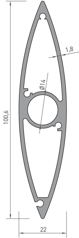
5437 GÜNEŞ KIRICI PROFİLİ 1,305 kg/mt Jx : 31,87 cm 4 Jy : 2,45 cm 4
