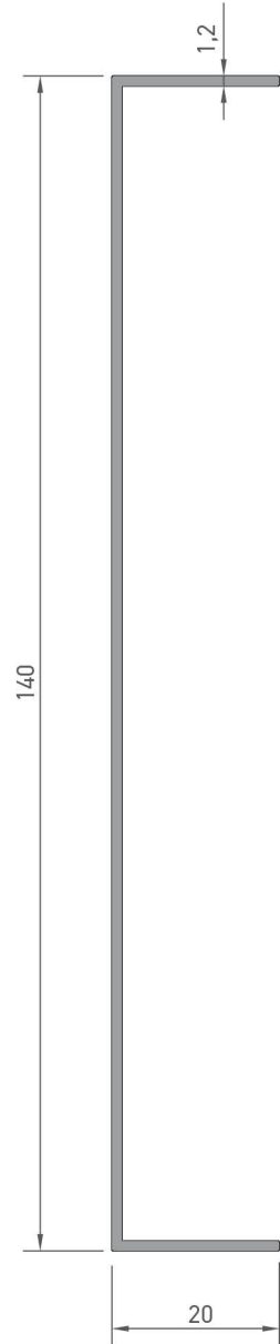
5430 GÜNEŞ KIRICI KASA PROFİLİ 0,580 kg/mt Jx : 49,15 cm 4 Jy : 0,50 cm 4
