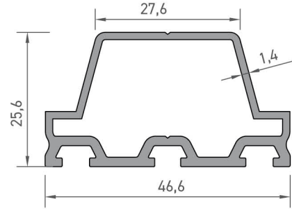
2493 ALT BAĞLANTI PROFİLİ 0,640 kg/mt
