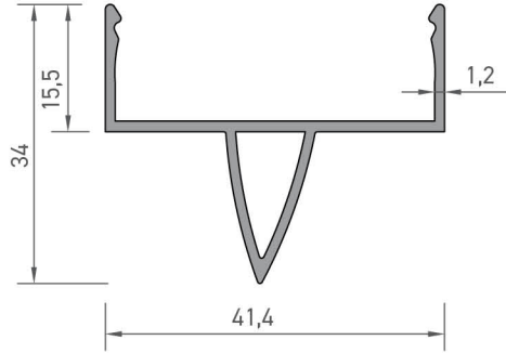
4586 ÇİTA PROFİLİ 0,365 kg/mt
