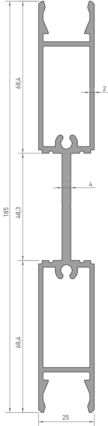
5494 KASA ORTA ROFİLİ (25'LİK) 2,775 kg/mt Jx : 8,35 cm 4 Jy : 295,36 cm 4
