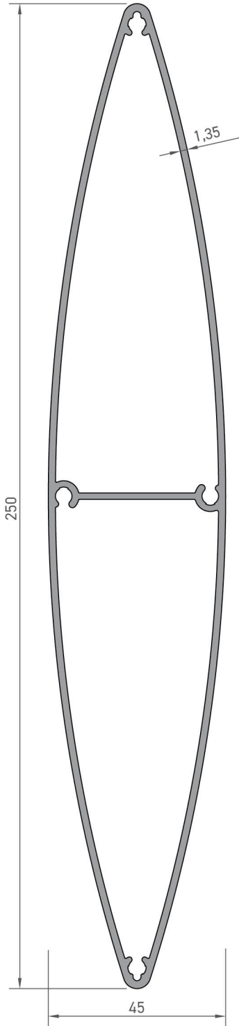
3845 GÜNEŞ KIRICI PROFİLİ 2,760 kg/mt Jx : 161,31 cm 4 Jy : 7,95 cm 4
