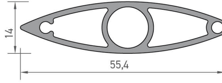
1954 YAPRAK PROFİLİ 0,560 kg/mt
