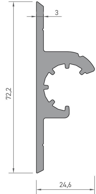
3763 BAĞLANTI PROFİLİ 1,125 kg/mt Jx : 10,99 cm 4 Jy : 1,54 cm 4
