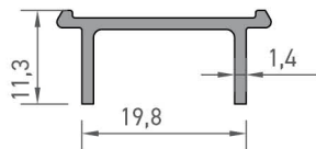
2484 ALT TUTAMAK PROFİLİ 0,170 kg/mt
