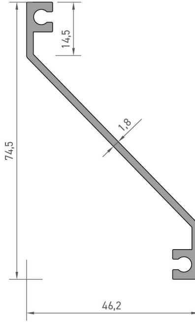
5439 GÜNEŞ KIRICI YAPRAK 0,590 kg/mt Jx : 18,31 cm 4 Jy : 0,23 cm 4
