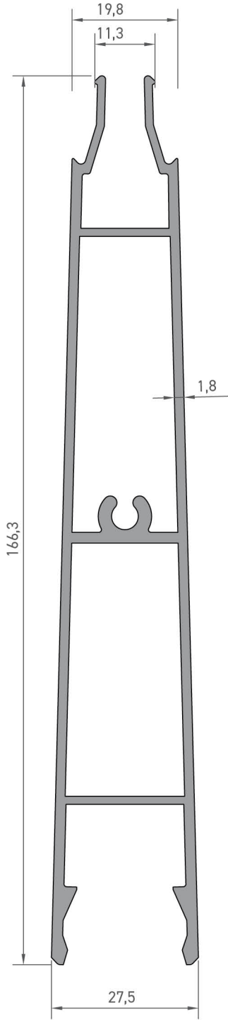
5497 GÜNEŞ KIRICI YAPRAK PROFİLİ 2,090 kg/mt Jx : 170,30 cm 4 Jy : 7,53 cm 4
