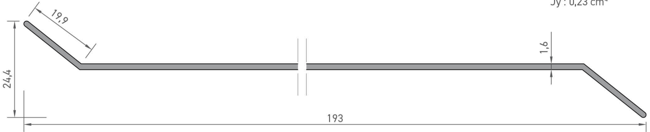
5434 GÜNEŞ KIRICI PROFİLİ 0,865 kg/mt Jx : 1,76 cm 4 Jy : 0,10 cm 4
