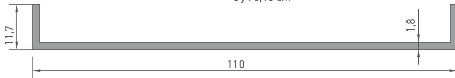
5435 GÜNEŞ KIRICI KASA PROFİLİ 0,635 kg/mt Jx : 30,40 cm 4 Jy : 0,14 cm 4
