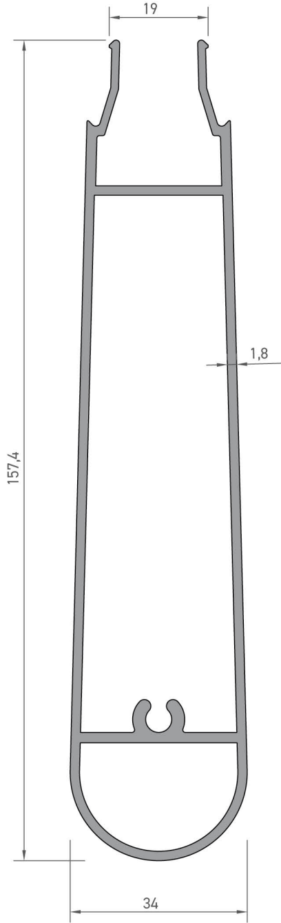
5496 GÜNEŞ KIRICI YAPRAK PROFİLİ 2000 kg/mt Jx : 168,76 cm 4 Jy : 11,87 cm 4
