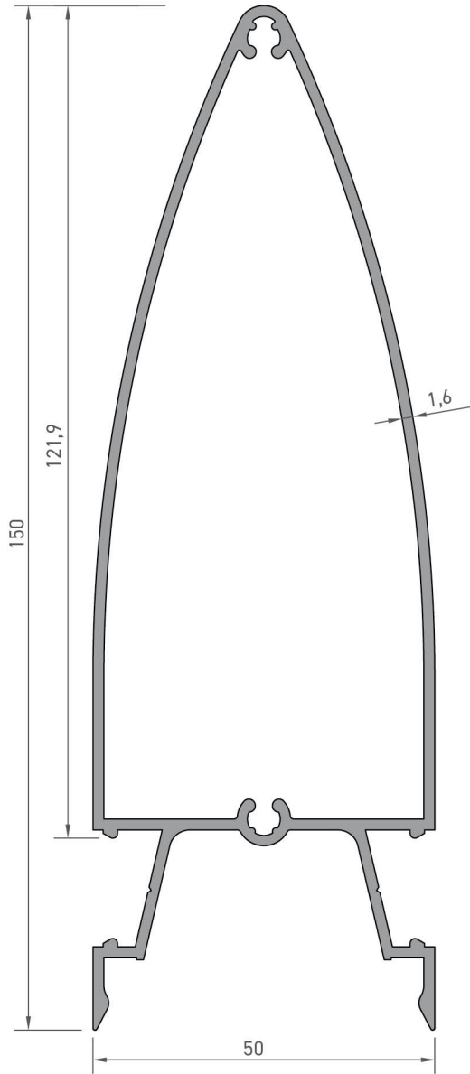
2492 ÜST KAPAK PROFİLİ 1,695 kg/mt Jx : 126,57 cm 4 Jy : 21,10 cm 4
