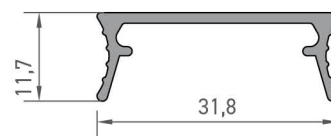
2485 TUTAMAK PROFİLİ 0,210 kg/mt
