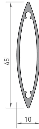
1973 GÜNEŞ KIRICI YAPRAK PROFİLİ 0,290 kg/mt Jx : 1,75 cm 4 Jy : 0,23 cm 4
