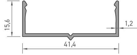
4585 HAREKETLİ ÇİTA PROFİLİ 0,250 kg/mt
