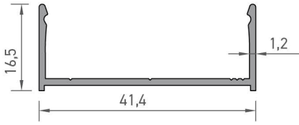
4377 SABİT ÇİTA PROFİLİ 0,245 kg/mt
