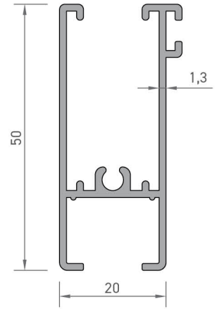
2305 TEK CAMLI KANAT ALT/ÜST PROFİLİ 0,550 kg/mt
