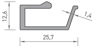
2319 KANAT RAY PROFİLİ 0,240 kg/mt
