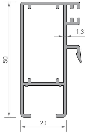
2304 TEK CAMLI KANAT ORTA PROFİLİ 0,625 kg/mt
