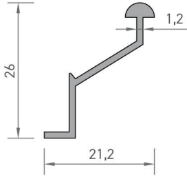
2308 SİNEKLİK RAY PROFİLİ 0,150 kg/mt
