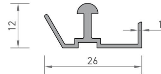
2307 KANAT RAY PROFİLİ 0,175 kg/mt
