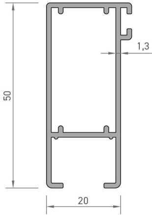
2303 TEK CAMLI KANAT YAN PROFİLİ 0,550 kg/mt
