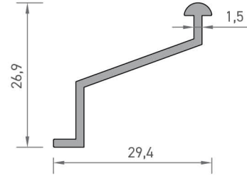
2309 SİNEKLİK RAY PROFİLİ 0,205 kg/mt
