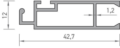
2311 SİNEKLİK PROFİLİ 0,375 kg/mt
