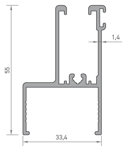
2317 ISI CAMLI KANAT ALT/ÜST PROFİLİ 0,700 kg/mt
