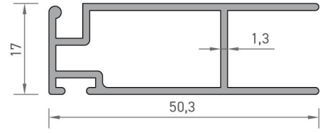
2313 SİNEKLİK PROFİLİ 0,505 kg/mt
