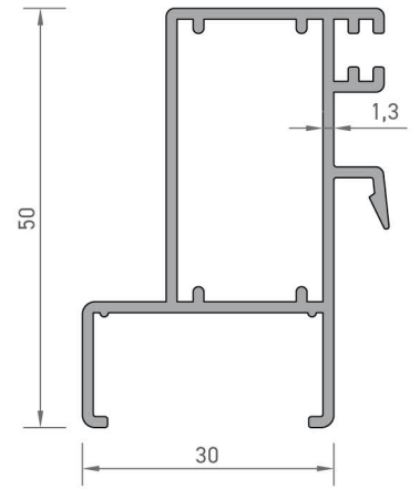
2301 ISI CAMLI KANAT ORTA PROFİLİ 0,650 kg/mt
