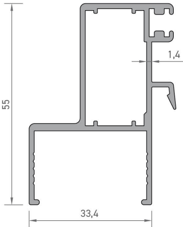
2318 ISI CAMLI KANAT ORTA PROFİLİ 0,765 kg/mt
