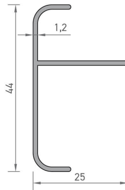
2320 KAPAMA PERVAZ PROFİLİ 0,265 kg/mt
