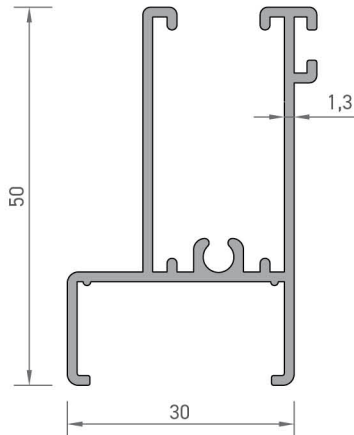
2300 ISI CAMLI KANAT ALT/ÜST PROFİLİ 0,570 kg/mt
