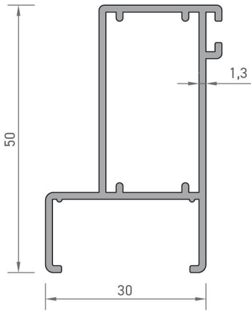
2302 ISI CAMLI KANAT YAN PROFİLİ 0,570 kg/mt
