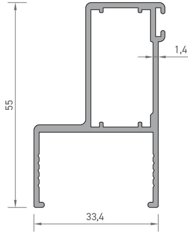
2316 ISI CAMLI KANAT YAN PROFİLİ 0,665 kg/mt
