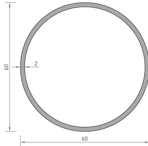
2860 BORU PROFİLİ 0,960 kg/mt
