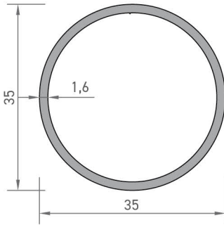
2498 BORU PROFİLİ 0,455 kg/mt
