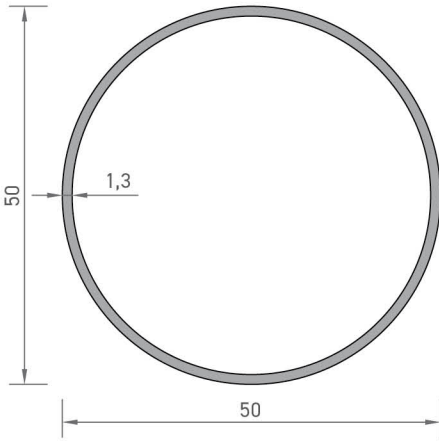
4652 BORU PROFİLİ 0,540 kg/mt
