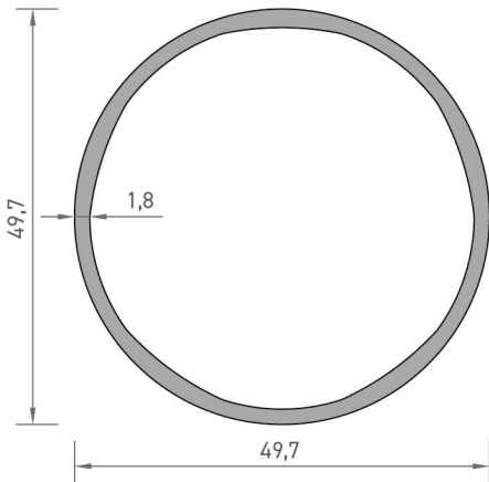
2463 BORU PROFİLİ 0,774 kg/mt
