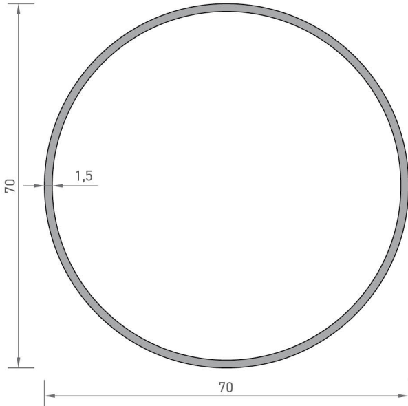
7551 BORU PROFİLİ 0,872 kg/mt
