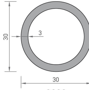
3020 BORU PROFİLİ 0,690 kg/mt
