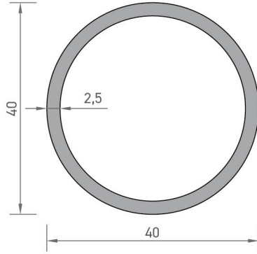
4958 BORU PROFİLİ 0,800 kg/mt
