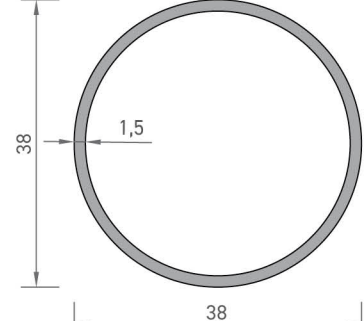
9130 BORU PROFİLİ 0,466 kg/mt
