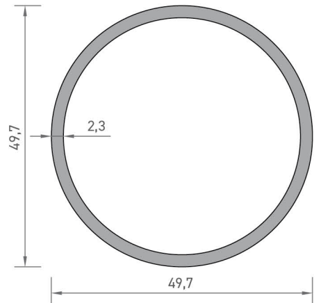
2455 BORU PROFİLİ 0,930 kg/mt
