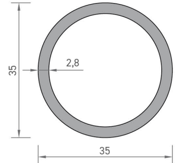
2462 BORU PROFİLİ 0,770 kg/mt
