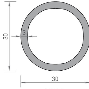
2461 BORU PROFİLİ 0,645 kg/mt
