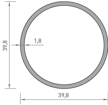
2865 BORU PROFİLİ 0,585 kg/mt
