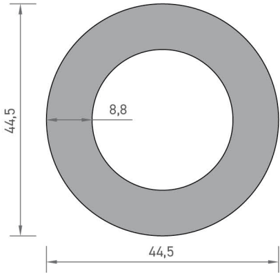
6784 BORU PROFİLİ 2,663 kg/mt
