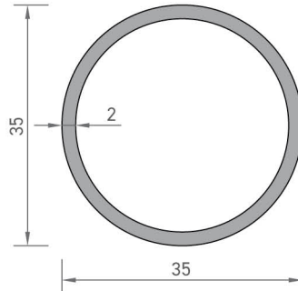
2467 BORU PROFİLİ 0,560 kg/mt
