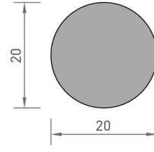
4819 DOLU BORU PROFİLİ 0,860 kg/mt
