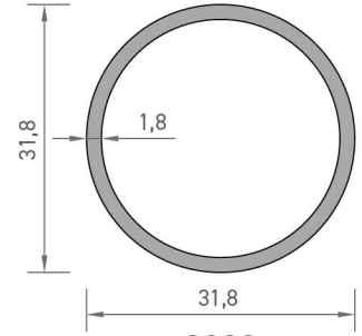
2982 BORU PROFİLİ 0,455 kg/mt
