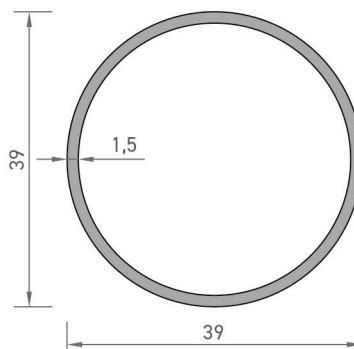
9170 BORU PROFİLİ 0,478 kg/mt
