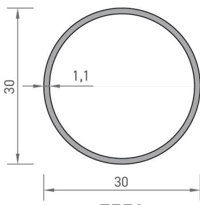
7552 BORU PROFİLİ 0,270 kg/mt
