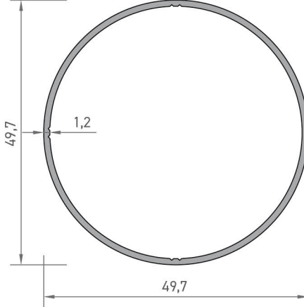
6101 BORU PROFİLİ 0,474 kg/mt
