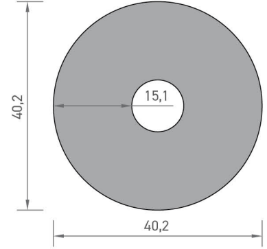
3017 BORU PROFİLİ 3,230 kg/mt
