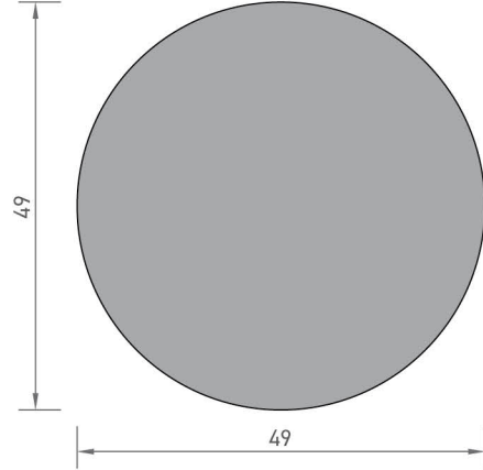
6130 DOLU BORU PROFİLİ 2,607 kg/mt
