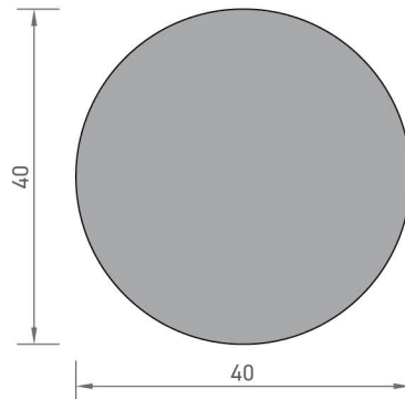
3012 DOLU BORU PROFİLİ 3,406 kg/mt
