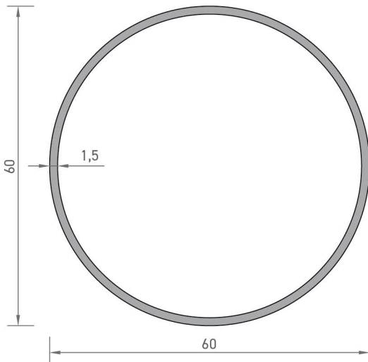
8008 BORU PROFİLİ 0,750 kg/mt
