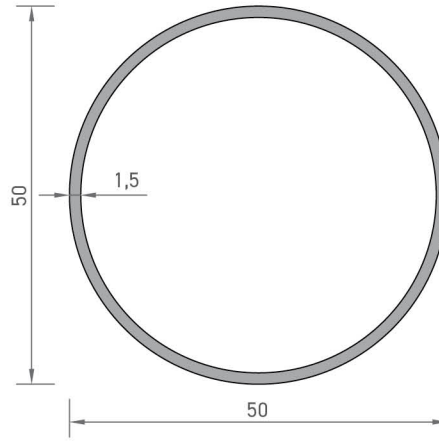
2466 BORU PROFİLİ 0,620 kg/mt
