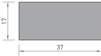
4867 DOLU KUTU PROFİLİ 1,717 kg/mt
