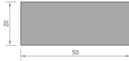
8517 DOLU KUTU PROFİLİ 2,710 kg/mt
