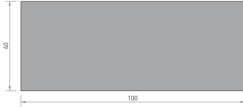
8552 DOLU KUTU PROFİLİ 10,840 kg/mt
