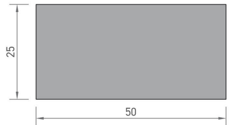
2897 DOLU KUTU PROFİLİ 2,439 kg/mt
