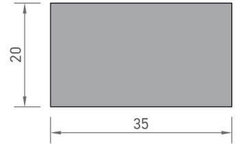
8484 DOLU KUTU PROFİLİ 1,897 kg/mt
