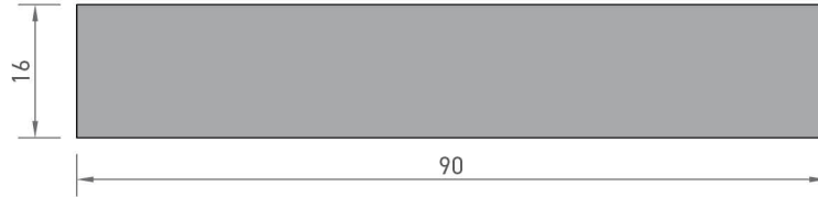
8737 DOLU KUTU PROFİLİ 3,903 kg/mt
