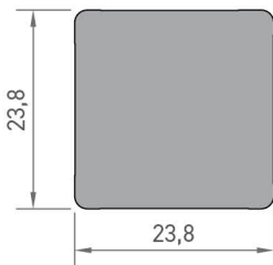
6208 DOLU KUTU PROFİLİ 1,536 kg/mt
