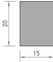
8599 DOLU KUTU PROFİLİ 0,813 kg/mt
