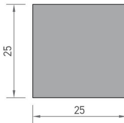
2894 DOLU KUTU PROFİLİ 1,694 kg/mt
