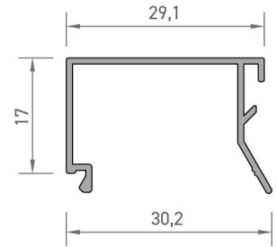
2104 TEK CAM ÇITA PROFİLİ (2144 NOLU PROFİL İÇİN) 0,190 kg/mt
