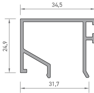
4636 KASA TEK CAM ÇITA PROFİLİ 0,430 kg/mt
