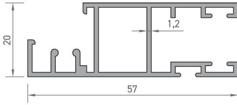
2133 SİNEKLİK KANAT PROFİLİ 0,605 kg/mt
