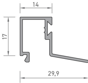
2105 ISI CAM ÇITA PROFİLİ (2144 NOLU PROFİL İÇİN) 0,230 kg/mt
