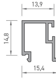
2138 ISI CAM ÇITA PROFİLİ (2149 NOLU PROFİL İÇİN) 0,175 kg/mt
