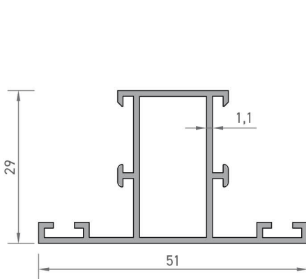
2258 ORTA KAYIT PROFİLİ 0,485 kg/mt
