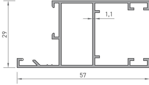
2132 DAR KANAT PROFİLİ 0,520 kg/mt
