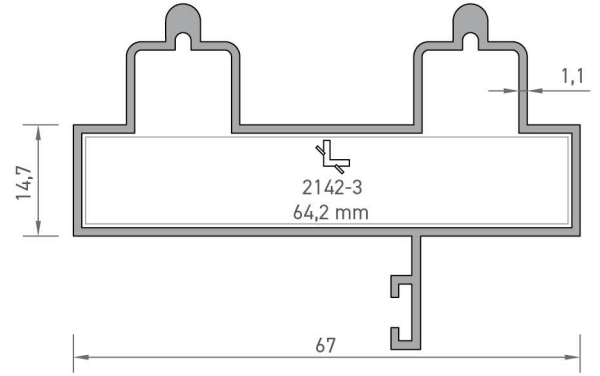
2139 BİNİLİ RAYLI KASA PROFİLİ 0,760 kg/mt
