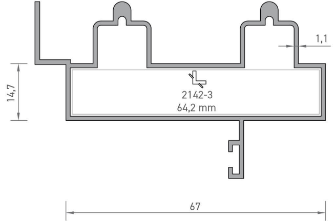
2128 OLUKLU RAYLI KASA PROFİLİ 0,840 kg/mt
