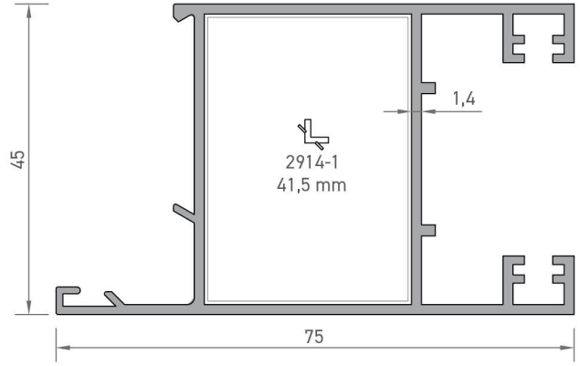
2144 GENİŞ KANAT PROFİLİ 1,065 kg/mt
