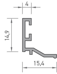
2136 ISI CAM ÇITA PROFİLİ 0,135 kg/mt
