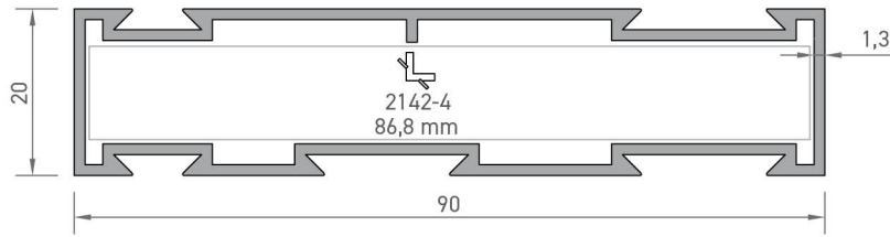
2140 SİNEKLİK KASA PROFİLİ 0,935 kg/mt
