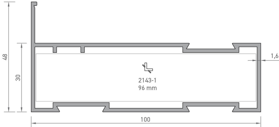
2150 KULAKLI GENİŞ KASA PROFİLİ 1,300 kg/mt
