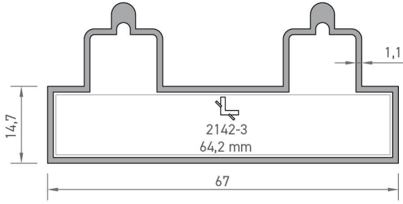
2119 RAYLI KASA PROFİLİ 0,690 kg/mt
