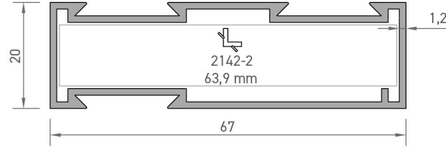
2130 DAR KASA PROFİLİ 0,685 kg/mt
