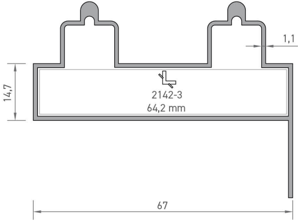
2188 KULAKLI RAYLI KASA PROFİLİ 0,655 kg/mt
