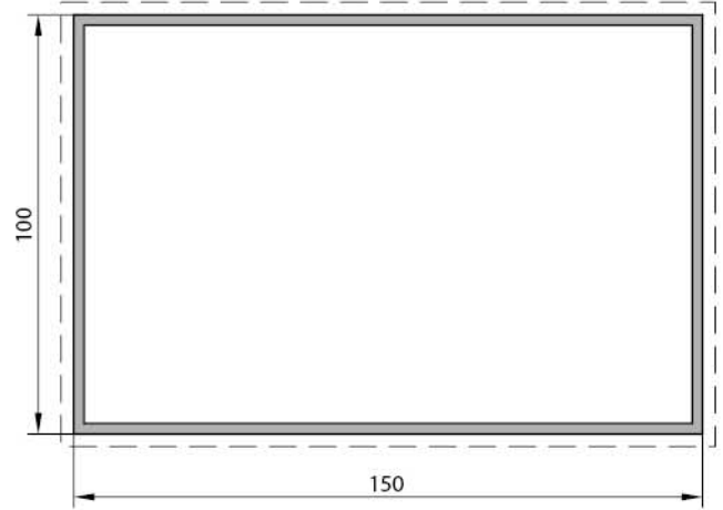
DİKME PROFILI V.SC.108 3.320 kg/mt
