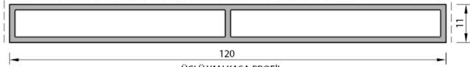
ÜÇLÜ YAN KASA PROFİL V.ES.101 1.065 kg/mt
