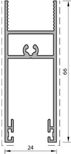
BAZA PROFİLİ V.E.S.261 0.761 kg/mt
