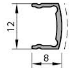
MOTOR KAPAK PROFİLİ 2458 0.065 kg/mt
