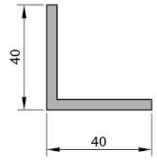
KÖŞE PROFILI V.SC.109 0.820 kg/mt
